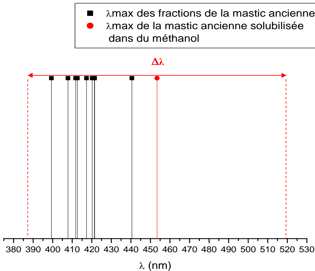
Figure 12 : Distribution de la longueur d'onde du maximum du spectre de fluorescence de chaque fraction issu de la séparation de la résine mastic ancienne (en noir) en comparaison avec la longueur d'onde du maximum et la largeur à mi hauteur du spectre de la résine solubilisée dans du méthanol (en rouge) ( \lambda_{\text{exc}}=320 nm)
