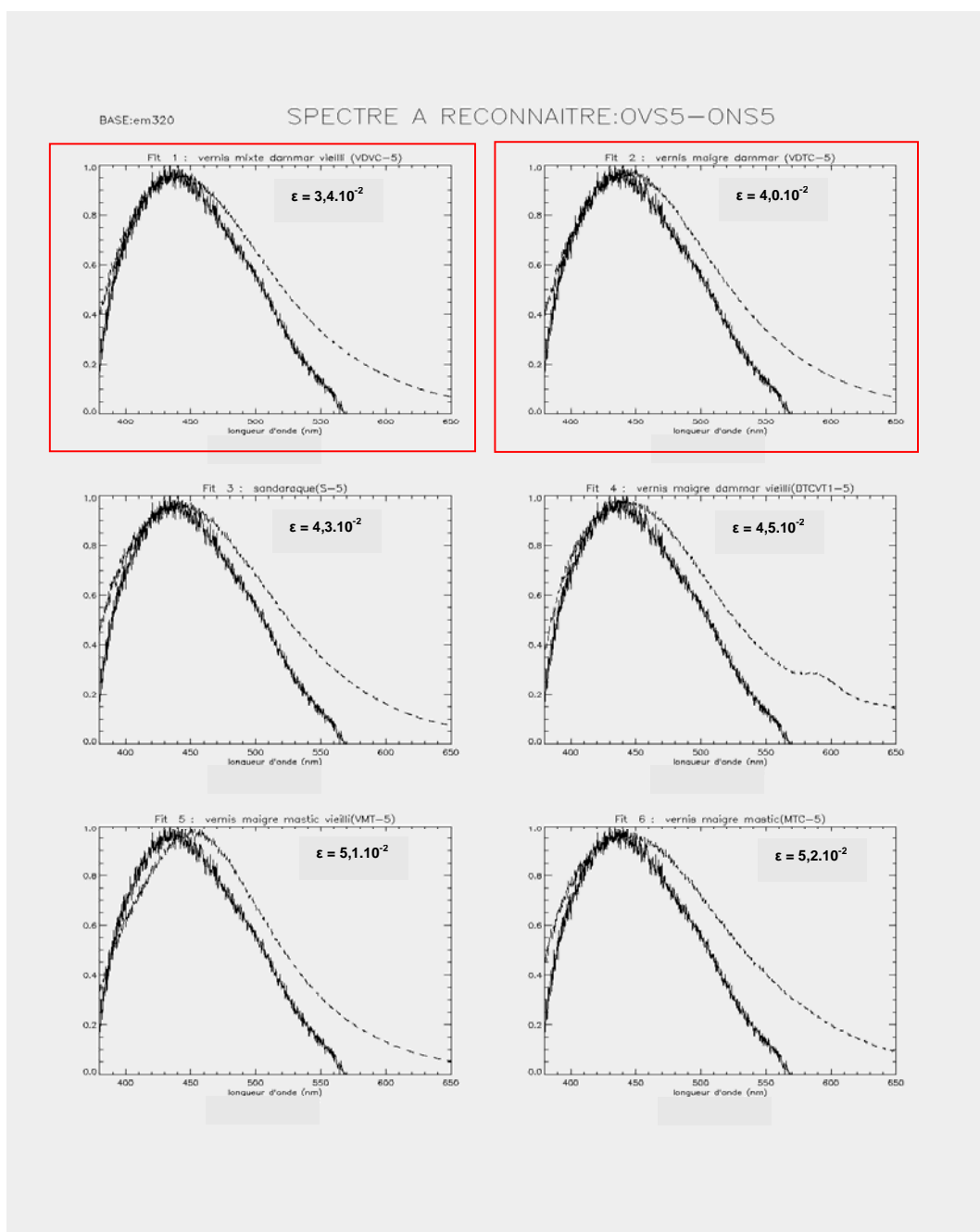
Figure 11 : Classement des six spectres de référence les plus concordant avec celui de la résine dammar du vernis apposé sur la couche picturale elle-même fluorescente ( \lambda_{exc} = 320 \text{ nm} .)
