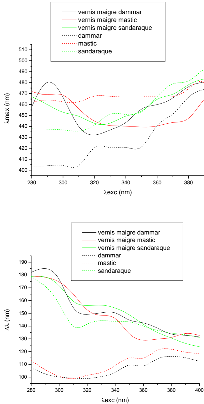
Figure 15 : variation de la longueur d'onde \lambda_{\max} du maximum et de la largeur à mi-hauteur \Delta\lambda des spectres des vernis maigres dammar, mastic et sandaraque frais comparés aux résines brutes correspondantes, en fonction de la longueur d'onde d'excitation \lambda_{\text{exc}}
