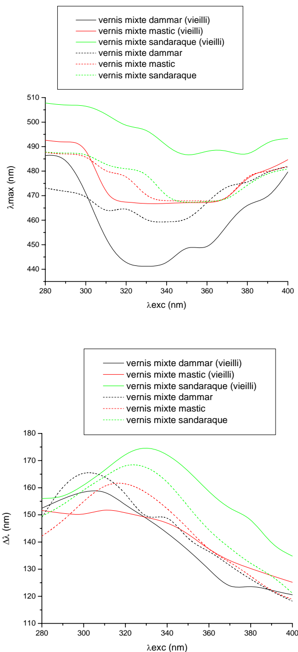
Figure 18 : variations de la longueur d'onde \lambda_{\max} du maximum et de la largeur à mi-hauteur \Delta\lambda des spectres des vernis mixtes dammar, mastic et sandaraque frais vieillis et frais en fonction de la longueur d'onde d'excitation \lambda_{\text{exc}}
