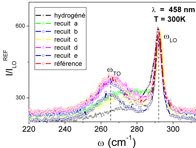
FIG. II.6 – Spectres Raman en configuration z(X, Y)\bar{z} , à T = 300 \text{ K} , sous laser Ar \lambda = 458 \text{ nm} . Pour faciliter la comparaison, les courbes ont été normalisées par rapport au pic du phonon LO de la référence. A basse densité de porteurs, le phonon LO domine, et sort à une valeur très proche de celle de la matrice hôte GaAs, \omega_{LO} = 292 \text{ cm}^{-1} . Lorsque p augmente, le mode couplé phonon LO-plasmon émerge progressivement, en se dirigeant vers la fréquence TO de la matrice hôte, \omega_{TO} = 267 \text{ cm}^{-1} .
