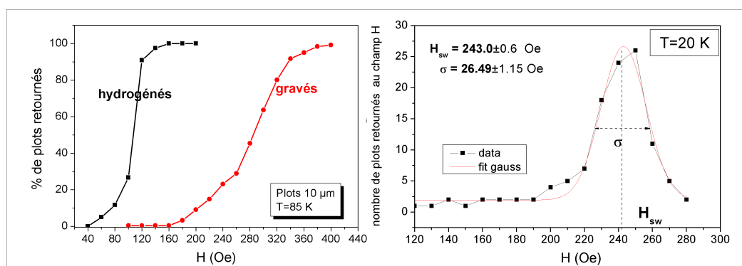
FIG. III.5 – (a) Renversement d’aimantation de plots hydrogénés et gravés de 10 \mu m de côté à 85 K. (b) Renversement d’aimantation de plots hydrogénés de 10 \mu m de côté à T=20 K. Détermination du champ moyen de retournement H_{sw} et de sa dispersion \sigma par ajustement à une gaussienne.
