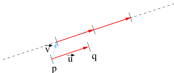
FIG. 3.7 – : Illustration des différentes définitions : un segment discret de vecteur directeur \vec{u} dans le premier octant, le vecteur de BEZOUT \vec{v} associé et les points de BEZOUT qui se trouvent sur la droite en pointillé et qui sont générés par \vec{u} .
