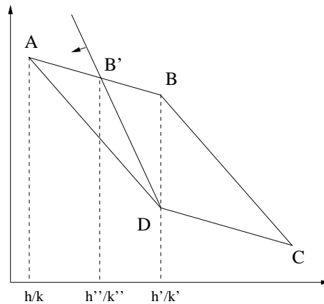
FIG. 2.17 –: L'ajout d'un nouveau point introduit une contrainte sur \bar{\mathcal{S}} d'ordre q , le point B' a une abscisse qui est le médian des abscisses de A et B dans la série de Farey d'ordre q + 1 .
