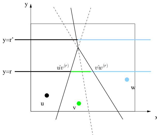
FIG. 4.5 —: Notations de BREU ET AL. : u , v et w sont des sites appartenant à P_r et P_{r'} , \hat{u}v^{(r)} et \hat{v}w^{(r)} sont les points intersections de la médiatrice de [uv] et [vw] respectivement, et de la droite y = r . Dans cet exemple, nous avons \mathcal{L}_r = \{u, v, w\} et \mathcal{L}_{r'} = \{u, w\} (voir le texte pour les explications).
