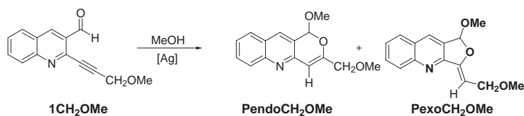
FIG. 6.3 – Réaction étudiée et nomenclature.
