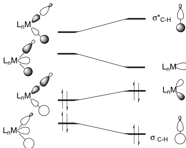
FIG. 8.10 – Diagramme de corrélation pour l'élimination réductrice de C-H
