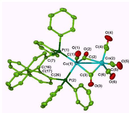
FIG. 7.3 – Structure cristallographique du \text{binap}(\text{PPh}_2)_2\text{Co}_2(\text{CO})_6
