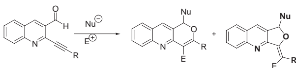
FIG. 6.1 – Bilan de la réaction tandem étudiée
