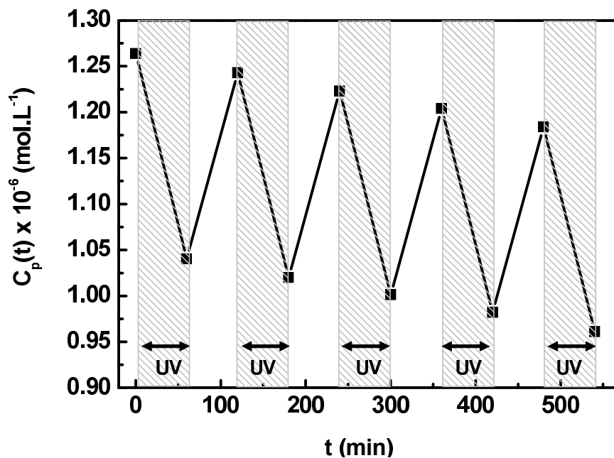
Figure VII-26 : Dégradation du BM avec insolation UV par alternance pour la membrane P70, T = 20°C, C a,0 = 1.10 -4 mol.L -1 .
