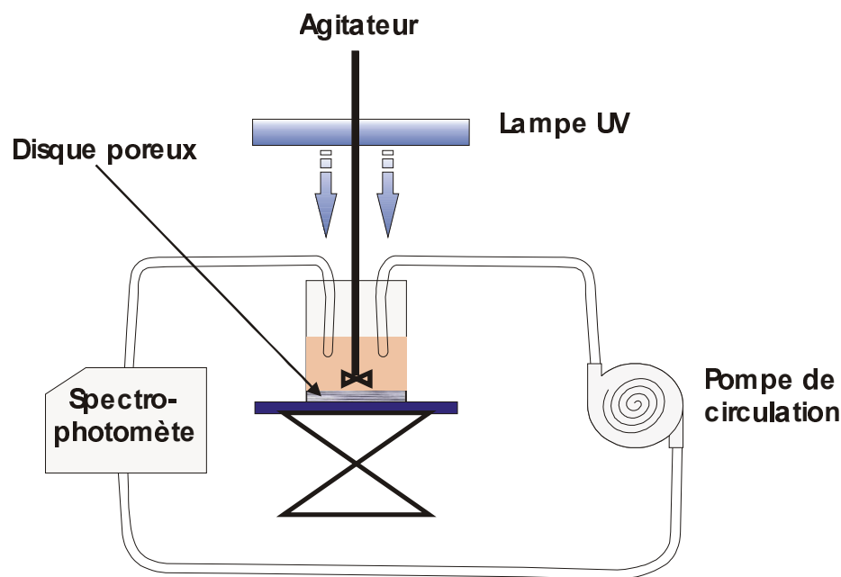
Figure VII-10 : Schéma de principe du dispositif expérimental.
