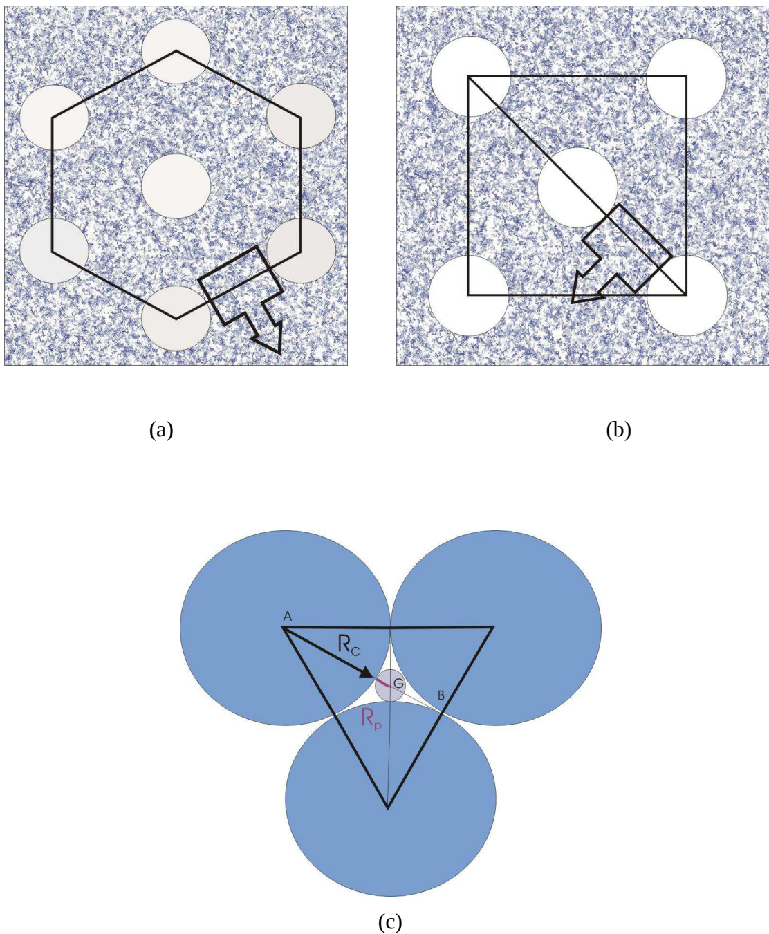
Figure VIII-12 : (a) Représentation schématique de l'arrangement des mésopores ordonnés dans la structure hexagonale 2D (P70), (b) Représentation schématique de l'arrangement des mésopores ordonnés dans la structure cubique (F67), (c) Représentation schématique de la porosité des murs de TiO 2 dans les zones de tangence des mésopores ordonnés ; avec R_c = L/2 , rayon des cristallites d'anatase et R_{p,géo} le rayon des pores correspondants.
