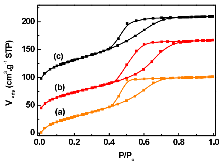
Figure VI-8 : Isothermes d'adsorption/désorption d'azote des poudres traitées à 350°C; (a) 50Ti : V_{50\text{Ti}} = V_{\text{ads}} + 50 , (b) 60Ti, (c) 45Ti : V_{45\text{Ti}} = V_{\text{ads}} - 40 .
