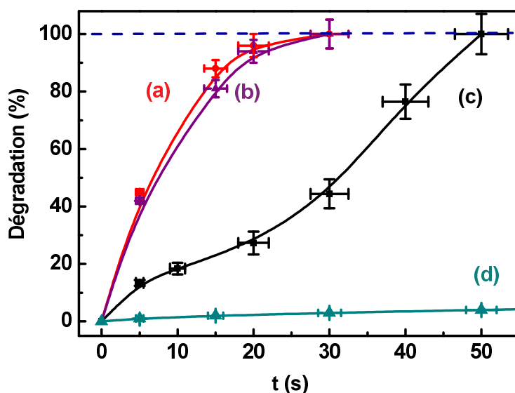
Figure VII-3 : Dégradation de l'acide stéarique en fonction de la durée d'irradiation sur différentes couches ;(a) P70, (b) F67, (c) bicouche sans ajout de copolymère, (d) référence sans dépôt de \text{TiO}_2 .
