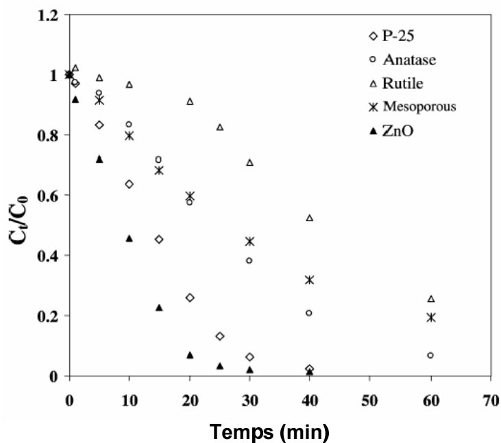
Figure I-2 : Comparaison entre la poudre P25 et différents matériaux photocatalytiques, d'après 32 .
