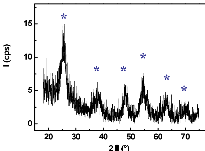
Figure VI-11 : Diffractogramme de \text{TiO}_2\text{-Ni} à 350^\circ\text{C} ; * anatase.
