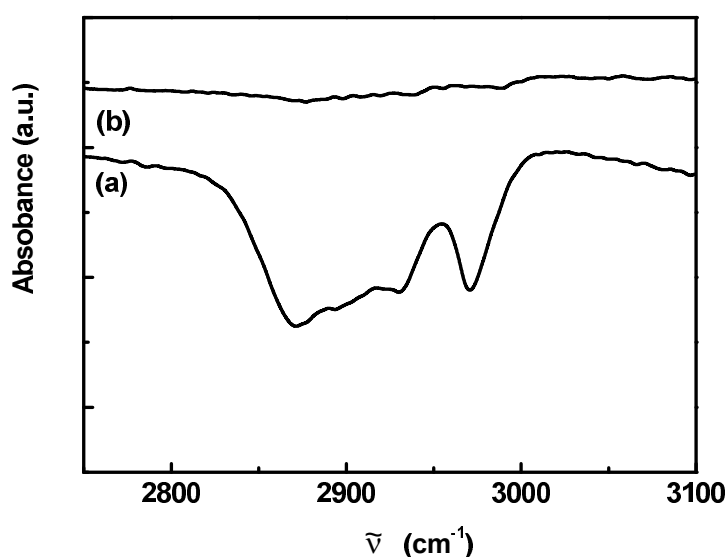
Figure V-6 : Evolution du spectre IR dans la gamme de vibration des \text{C-H} du P123 de la couche avant (a) et après (b) traitement UV d'une minute par face.
