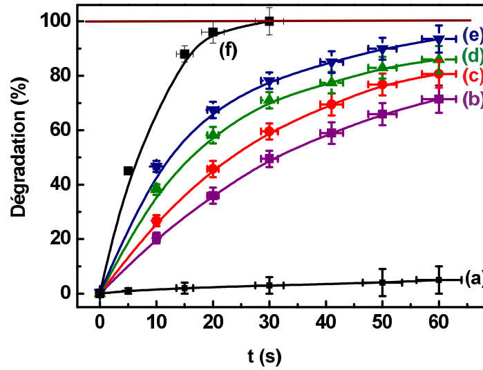
Figure VII-4 : Dégradation sur des couches mixtes \text{TiO}_2\text{-SiO}_2 – courbes brutes ; (a) référence sans couche de \text{TiO}_2 , (b) 50%, (c) 60%, (d) 70%, (e) 80%, (f) 100%.
