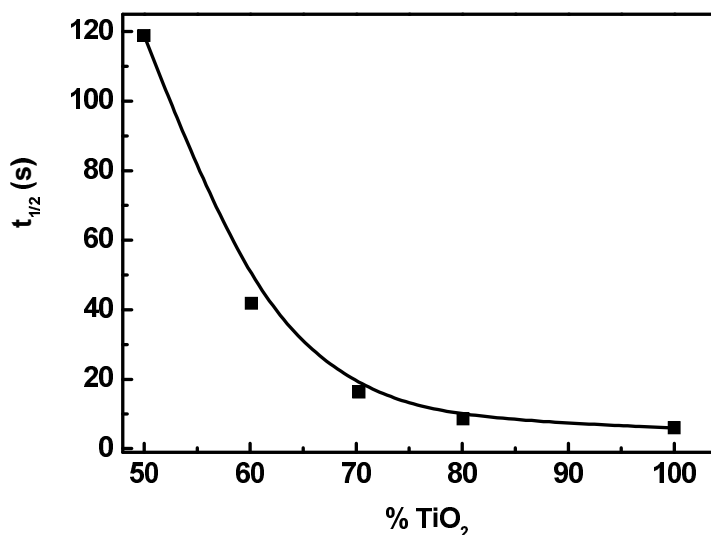
Figure VII- 6 : Evolution de t_{1/2} en fonction de la teneur en \text{TiO}_2 (données corrigées).
