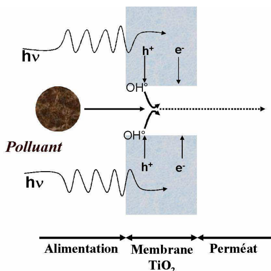
Figure II-13 : Schéma du concept de réaction photocatalytique dans un système de filtration 15 .
