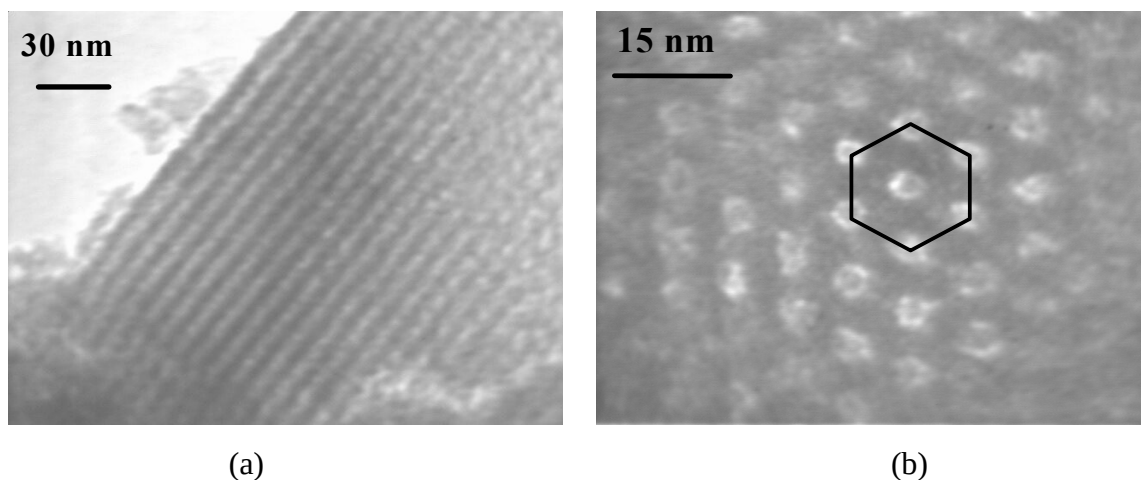
Figure V-10 : Images MET de la couche P70 à 25°C ; (a) dans le plan des micelles cylindriques, (b) perpendiculaire au plan des micelles cylindriques.
