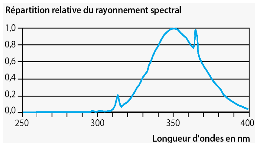
Figure VII-11 : Spectre d'émission de la lampe UV utilisée.
