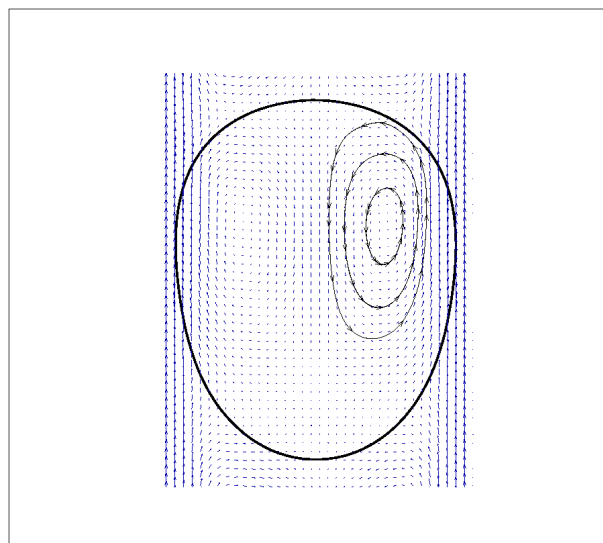
FIG. 8.14 – Petite goutte (trait noir), champ de vitesse associé dans le référentiel de la goutte (flèches bleues) et quelques lignes de courant (lignes fléchées) ; données de référence sauf que les viscosités dans la goutte et de la phase continue sont échangées.
