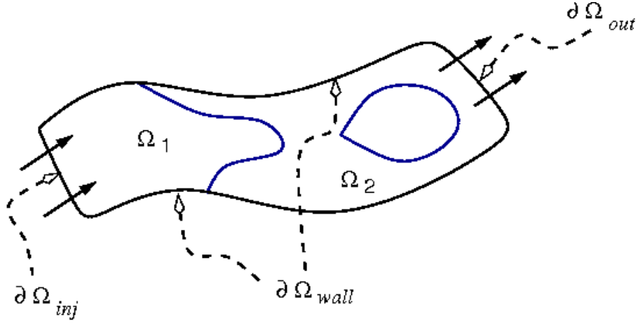
FIG. 5.2 – Partitionnement du bord de \Omega pour affecter différentes conditions aux limites.
