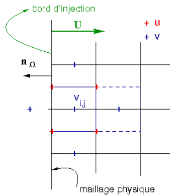
FIG. 5.10 – Maille en v tangente au bord d'injection
