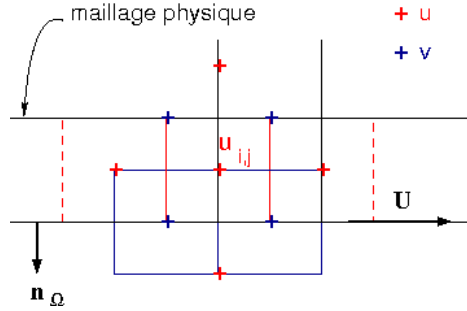
FIG. 5.9 – Maillage en u tangente à une paroi horizontale
