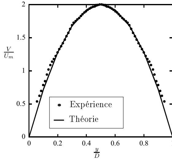
FIG. 2.10 – Profil de la vitesse du fluide adimensionnée par la vitesse moyenne en fonction de la hauteur adimensionnée par le diamètre du tube.
