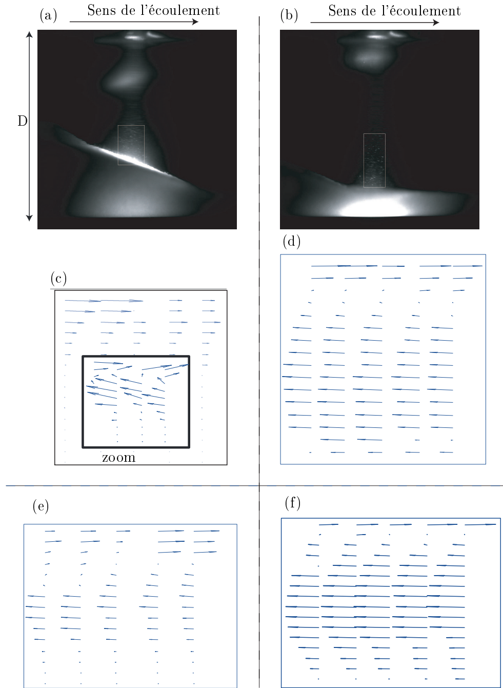
FIG. 5.6 – (a) et (b) Région où l'écoulement a été mesuré par PIV, (c) et (d) écoulement mesuré au centre du tube et (e) et (f) écoulement mesuré à 1 cm du bord du tube. Le carré blanc représente la partie de l'écoulement mesuré par PIV.
