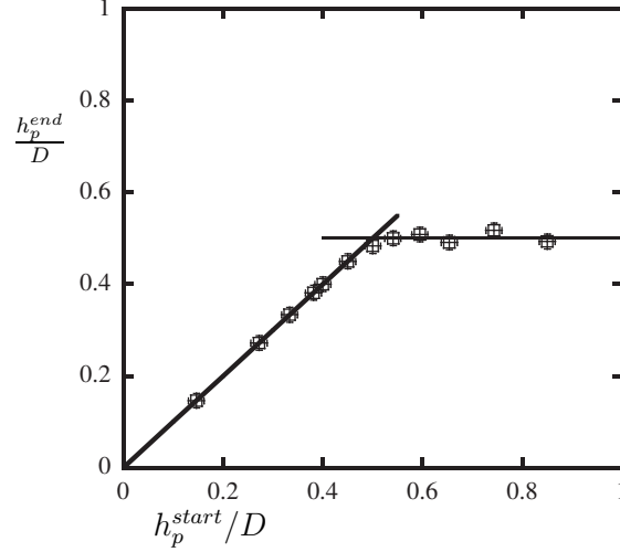
FIG. 3.2 – Évolution de h_p^{end} en fonction de h_p^{start} pour un débit fixé Q_{pipe} = (2.77 \pm 0.09)10^{-5}\text{m}^3/\text{s} pour des billes de type B dans le fluide 2.
