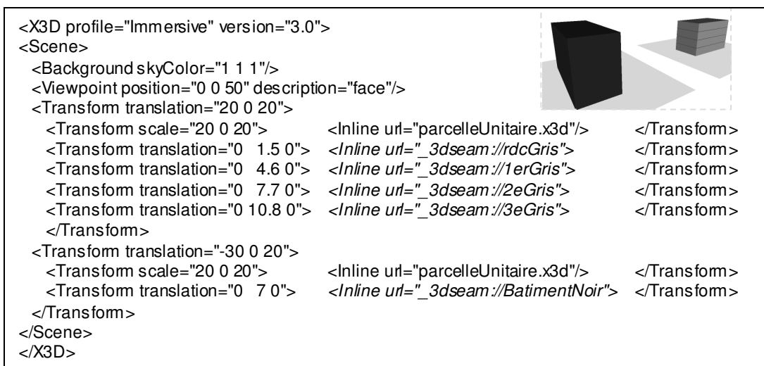
Figure 7.12 Pseudo description d'une scène 3D.
