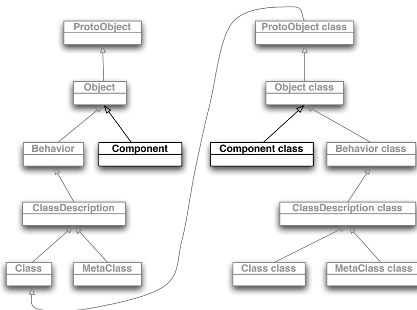
FIG. 5.2 : Implémentation actuelle du noyau de SCL
