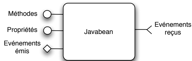
FIG. 2.9 : Structure d'un composant Javabean
