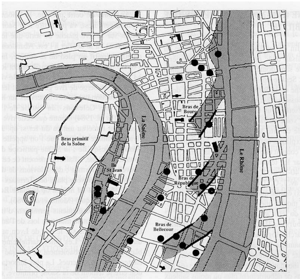
Fig. 16 – Restitution tracé de la confluence du Rhône et de la Saône à Lyon (BRAVARD 1995)
