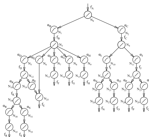
FIG. III.22 – Réseau neuro-flou de la zone surveillée
