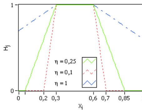
FIG. III.12 – Technique Fuzzy Min-Max - Sensibilité de l'hyper-cube
