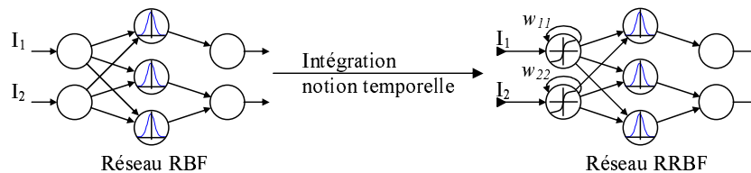
FIG. II.15 – Réseaux RFR et RRFR.
