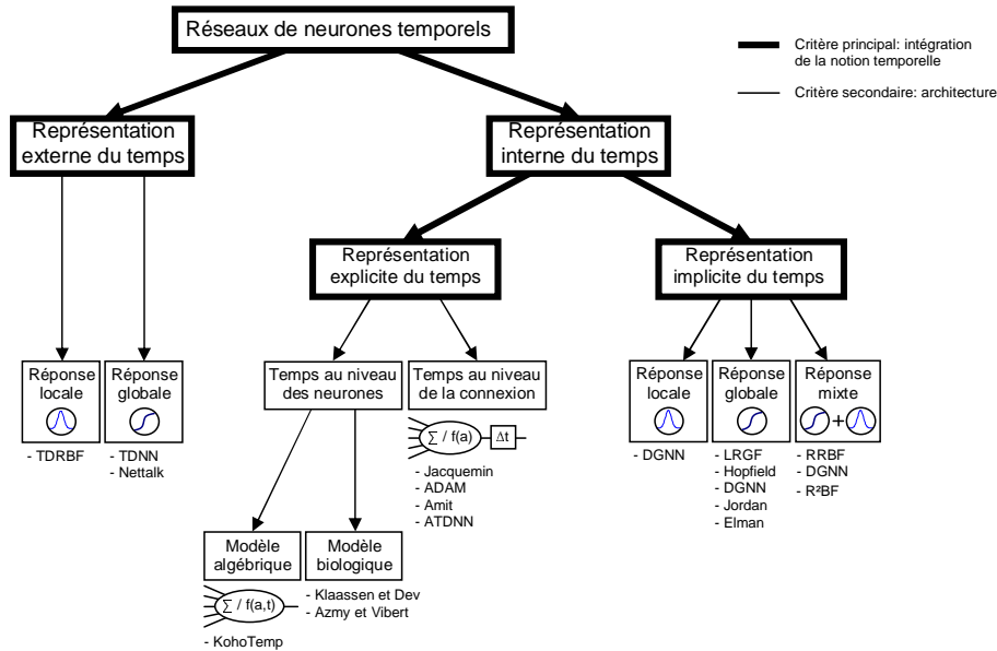
FIG. II.14 – Classification des réseaux de neurones temporels à l’aide de deux critères (temporel et architectural)
