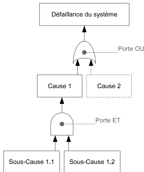
FIG. III.16 – Exemple d'arbre de défaillances
