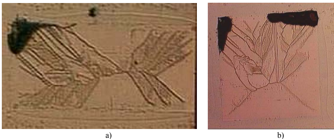
Fig. II. 3 : Vues de dessus en optique, a) motif de 2\text{mm}^2 et b) motif de 1\text{mm}^2 , présentant de nombreuses contraintes résiduelles après recristallisation. Le cycle de recristallisation utilisé est de 8\text{V}/2\text{s}/0\text{s} , l'épaisseur de silicium est de 13\mu\text{m} , et la couche d'encapsulant est 600\text{ \AA} de nitrure et 1,9\mu\text{m} d'oxyde déposé.
