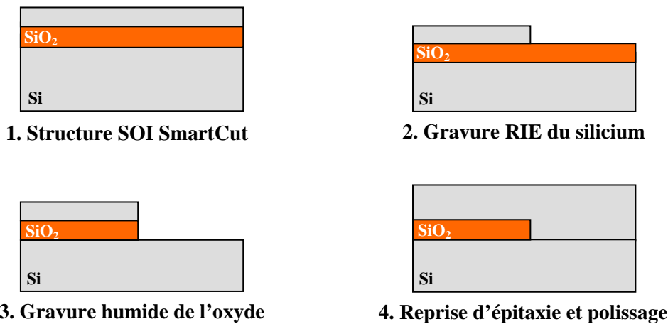
Fig. I.36 : Définition de substrats SOI partiel à partir de wafers SOI pleine plaque de type SmartCut ® .
