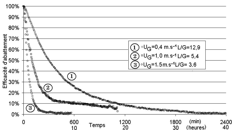
Figure III- 18 : Influence de la vitesse de gaz sur les courbes d'efficacité en fonction du temps ( L = 6,58 \text{ kg.s}^{-1}.\text{m}^{-2} )
