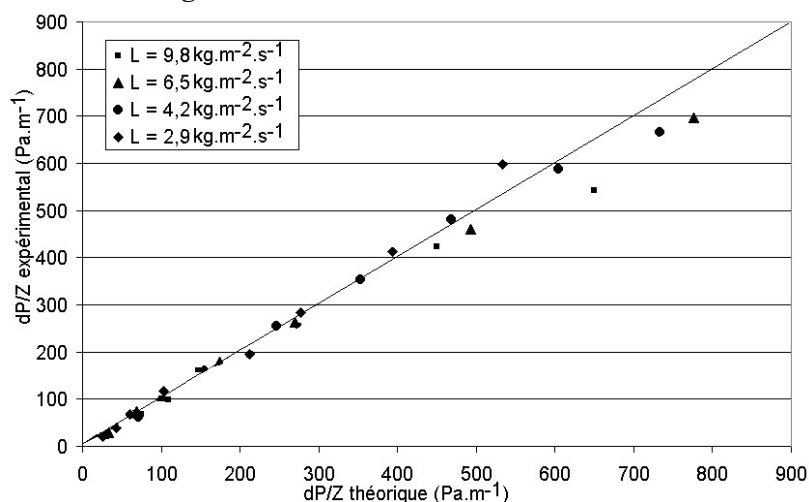
Figure III- 16 : Graphe de parité de la relation de Mackowiac concernant les pertes de charge en colonne arrosée
