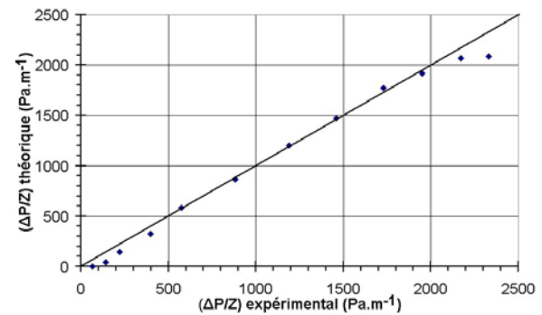
Figure A2-2 : Graphe de parité du modèle de Takahashi et Miyahara
