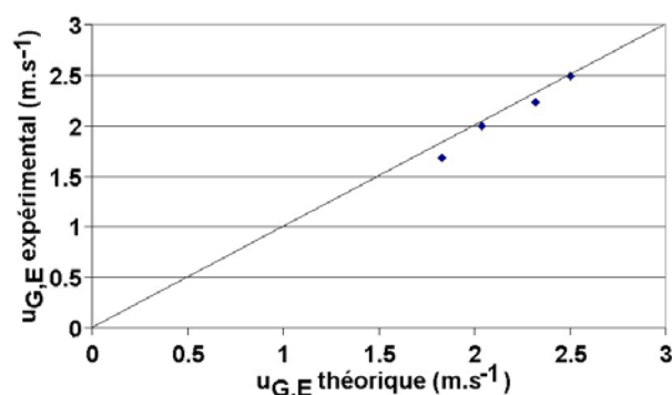
Figure III- 14 : Graphe de parité de la corrélation de Mackowiac concernant les vitesses de gaz à l'engorgement
