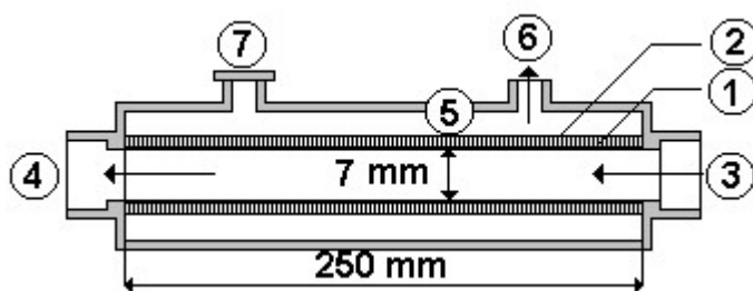
Figure IV- 5 : Module de pervaporation tubulaire
