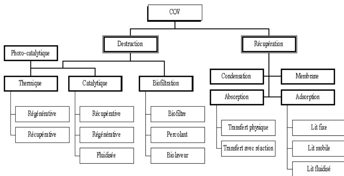
Figure I- 2 : Organigramme simplifié de différents procédés de traitement des COV 11
