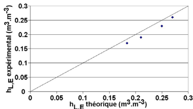
Figure III- 15 : Graphe de parité de la corrélation de Mackowiac concernant les rétentions de liquide à l'engorgement
