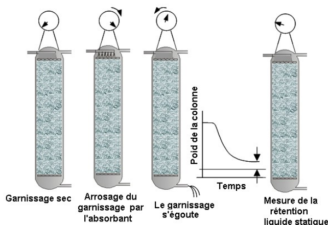
Figure III- 6 : Mesure de la rétention statique
