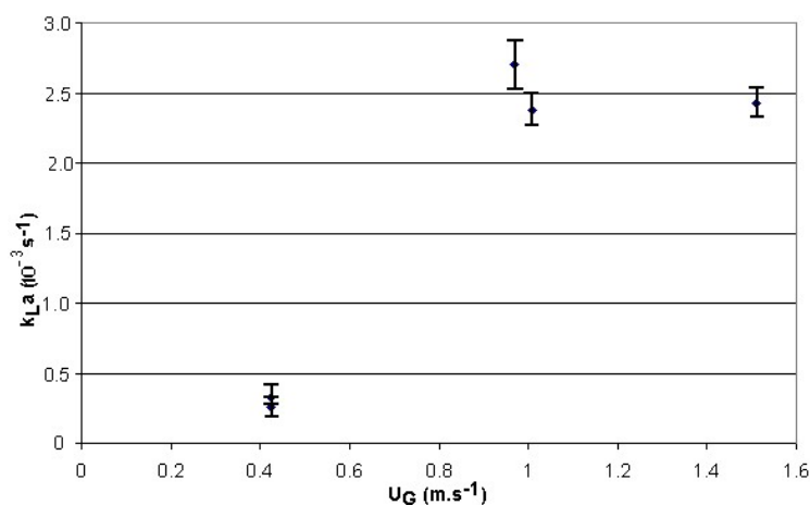
Figure III- 25 : Influence de la vitesse de gaz à débit de liquide fixé sur le k_{La}
