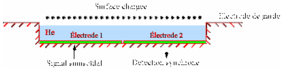
figure 39: Schéma du dispositif de détection des électrons dans l'expérience de Sommer et Tanner. L'électrode de garde confine les électrons au-dessus des électrodes 1 et 2. Une tension sinusoïdale est appliquée sur l'électrode 1. Le couplage capacitif entre les deux électrodes est mesuré par détection synchrone sur l'électrode 2. La présence des électrons augmente le couplage capacitif entre les deux électrodes.
