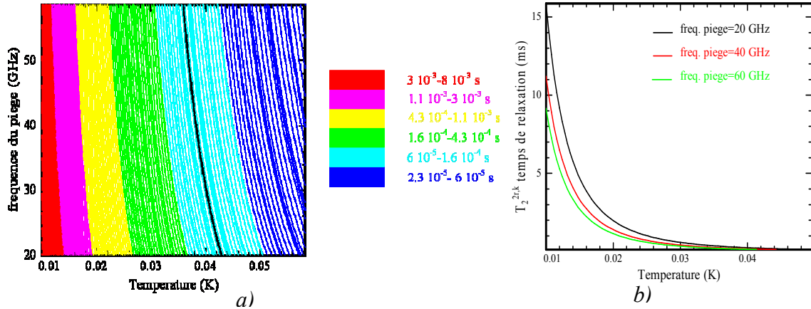
Figure 20 : a) évolution du temps de déphasage (cinétique+polarisation) en fonction de la température et de la fréquence d'oscillation. La ligne noire caractérise un temps de déphasage égal à 10 \mu s. b) pour trois valeurs d'oscillations différentes
