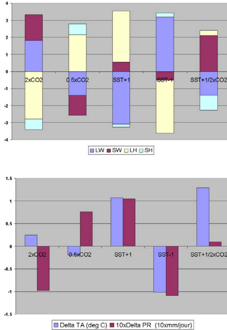
FIG. 2.5: Réponse du MCGA ARPEGE en moyenne globale au forçage par des anomalies radiatives, diabatiques ou combinées. 2xCO2 (0.5xCO2) correspond à un doublement (division par 2) de la concentration en CO 2 à TSO climatologique fixée. SST+1 (SST-1) correspond à une augmentation (diminution) des TSO climatologiques de 1 K à concentration en CO 2 fixée. SST+1/2xCO2 correspond à une expérience croisée où les deux perturbations sont appliquées. Pour le bilan énergétique, les valeurs positives (négatives) correspondent à un gain (perte) pour l'atmosphère (Wm -2 ). LH est le flux de chaleur latente, SH le flux de chaleur sensible, LW le bilan infrarouge net de l'atmosphère et SW le bilan solaire net de l'atmosphère. TA est la température de l'air en surface et PR les précipitations.
