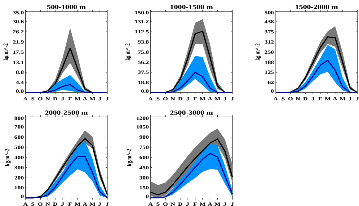
FIG. 11.24: Cycle saisonnier de la quantité d'eau du manteau neigeux ( \text{kg.m}^{-2} ) dans les Pyrénées par tranches d'altitude de 500 m pour le climat présent (1970/1999, gris et noir) et le climat futur (2046/2065 bleu clair et bleu foncé). La zone colorée est délimitée par les valeurs maximales et minimales des 14 modèles pour chaque mois, les traits épais sont les moyennes d'ensemble.
