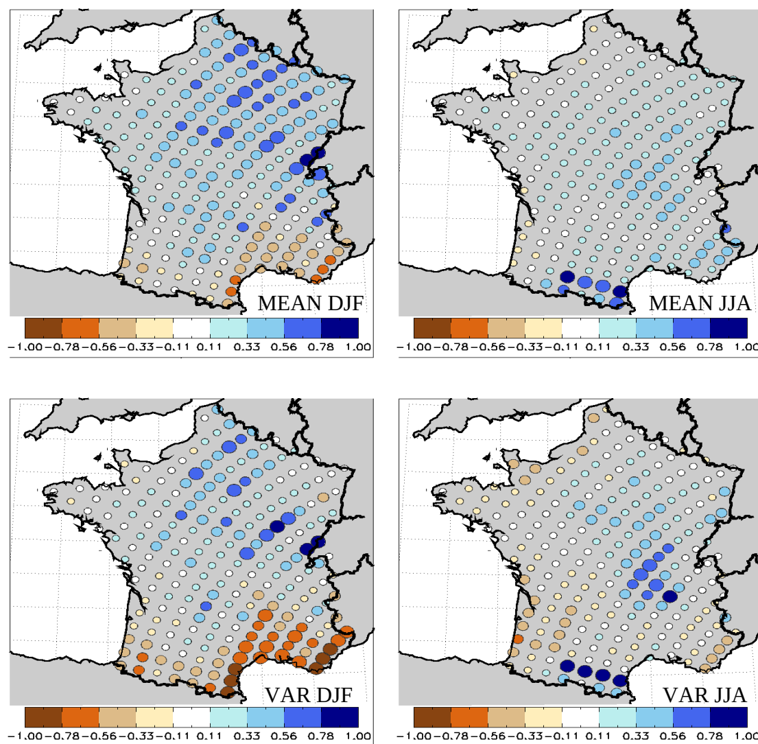
FIG. 7.3: Erreur relative pour la moyenne (MEAN, en haut) et la variance (VAR, en bas) des précipitations ARPEGE-VR sur la période 1971-1999 par rapport à l'analyse SAFRAN, en hiver (à gauche) et en été (à droite)
