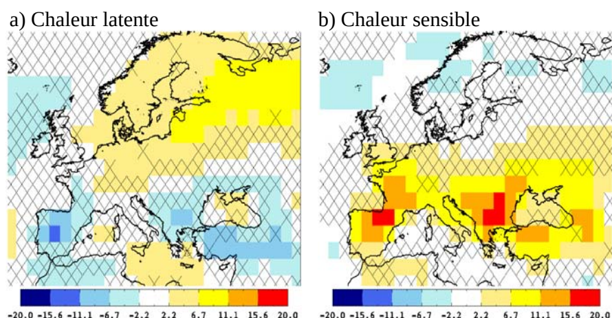
FIG. 10.18: Idem que Figure 10.15 pour (a) le flux de chaleur latente ( \text{W.m}^{-2} ) et (b) le flux de chaleur sensible ( \text{W.m}^{-2} ). Les flux sont comptés positivement vers le haut, un changement positif correspond donc à une perte d'énergie pour la surface.
