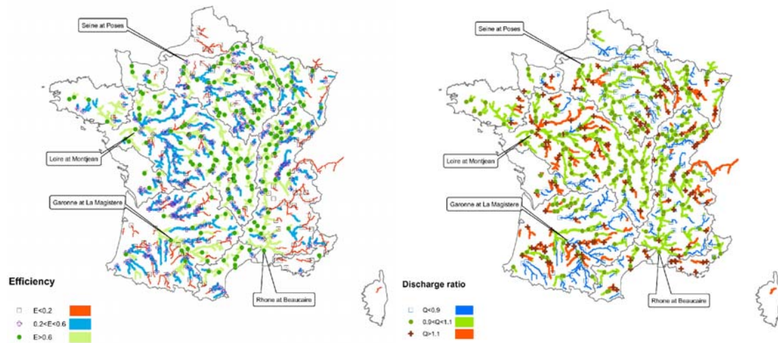
FIG. 4.4: Diagnostics de validation des débits simulés par SIM sur la période 1995-2005. A gauche, efficacité de Nash ; à droite, ratio des débits moyens simulés et observés. Source : Habets et al., 2007 .
