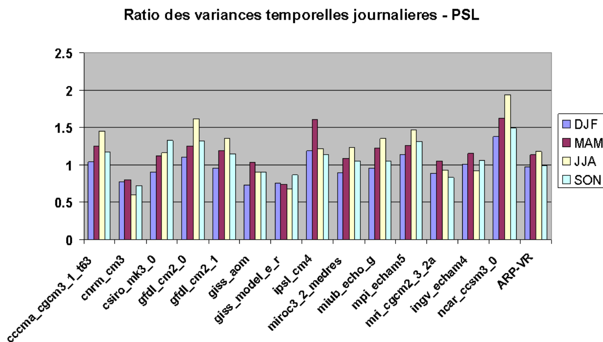
FIG. A.3: Moyenne spatiale du ratio des variances journalières de PSL (ratio inférieur à 1 : sous-estimation de la variance dans le modèle).
