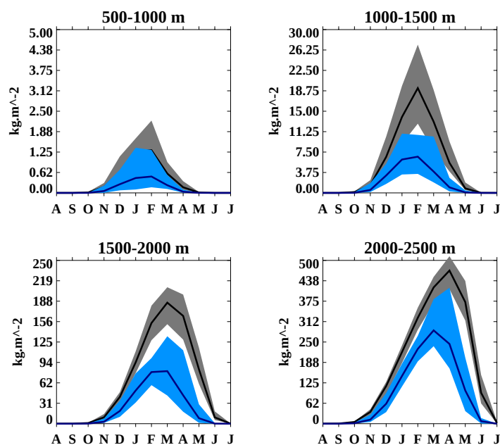
FIG. 11.24: Cycle saisonnier de la quantité d'eau du manteau neigeux ( \text{kg.m}^{-2} ) dans les Pyrénées par tranches d'altitude de 500 m pour le climat présent (1970/1999, gris et noir) et le climat futur (2046/2065 bleu clair et bleu foncé). La zone colorée est délimitée par les valeurs maximales et minimales des 14 modèles pour chaque mois, les traits épais sont les moyennes d'ensemble.
