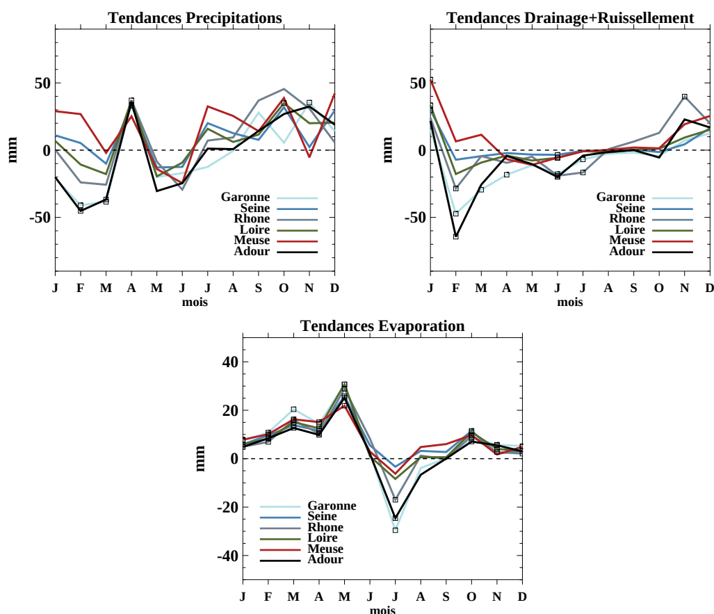
FIG. 4.12: Tendances mensuelles calculées sur la période 1970-2005 des précipitations, du ruissellement total et de l'évaporation (mm) en moyenne sur six principaux bassins versant français (le bassin de l'Adour et de la Meuse sont considérés ici en plus des 4 principaux bassins déjà mentionnés). Les tendances significatives à 0.05 sont marquées par des carrés.
