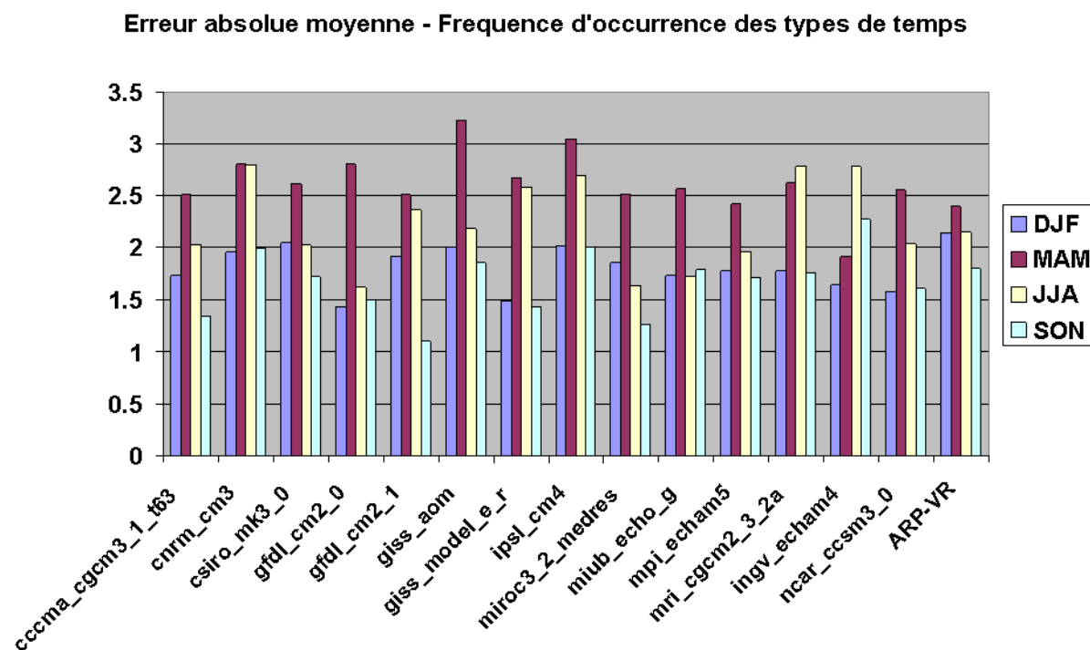
FIG. A.4: Erreur absolue moyenne sur la fréquence d'occurrence des types de temps de chaque saison (%).
