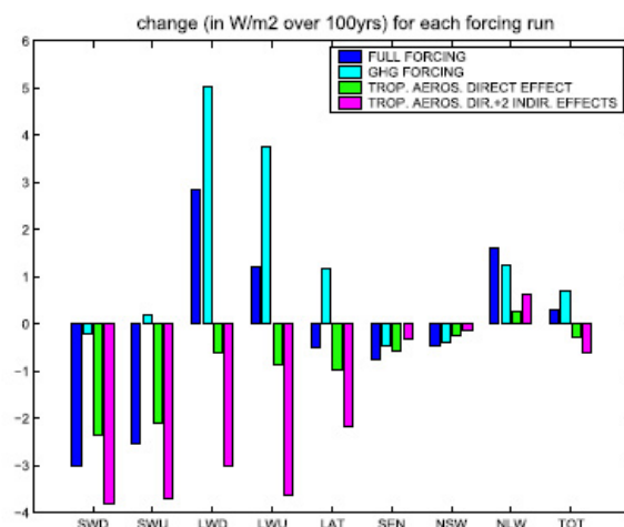
FIG. 2.10: Tendances linéaires ( \text{W/m}^2 sur 100 ans) pour 4 expériences de sensibilité (modèle climatique GISS-ER). La période simulée est le 20 ème siècle, avec différents forçages (GES uniquement, effet direct des aérosols troposphériques, effet direct + les 2 effets indirects des aérosols troposphériques, tous les forçages précédents réunis). SWD : downward shortwave radiation (positif vers le bas), SWU : upward shortwave (positif vers le haut), LWD : downward longwave (positif vers le bas), LWU : upward longwave (positif vers le haut), LAT : latent heat flux (positif vers le haut), SEN : sensible heat flux (positif vers le haut), NSW : net shortwave (positif vers le bas), NLW : net longwave (positif vers le bas), TOT : bilan énergétique total. Source : Romanou et al., 2007 .
