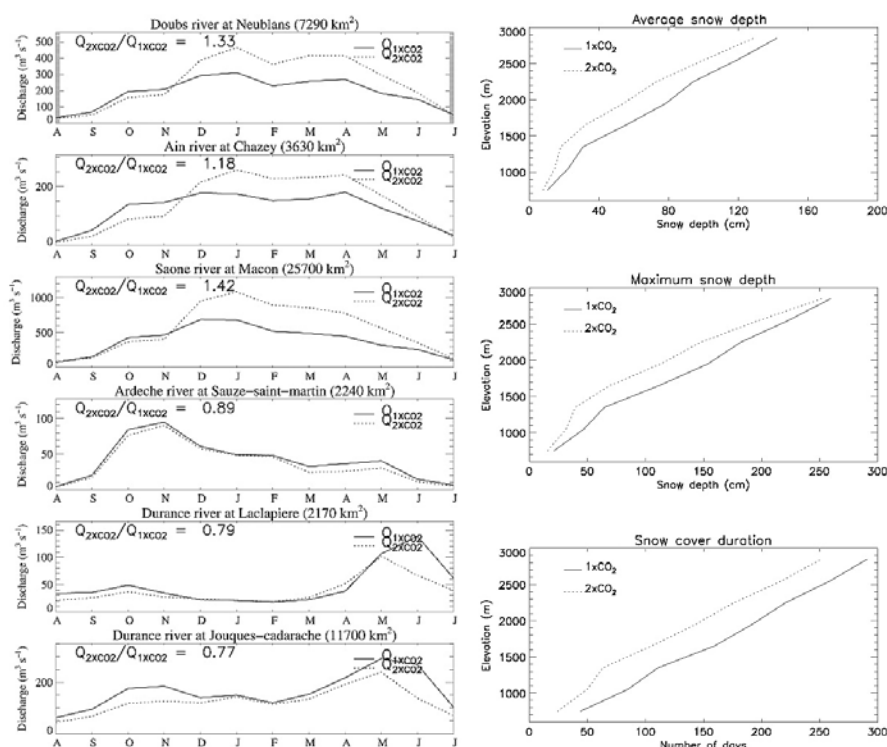
FIG. 3.6: Gauche : Débits mensuels de cours d'eau du bassin du Rhône, moyennés sur 14 années pour le climat actuel et pour un climat futur au taux de CO 2 doublé par rapport à la période pré-industrielle. Droite : Principales caractéristiques du couvert neigeux sur le bassin du Rhône pour le climat présent et pour le climat futur en fonction de l'altitude. Source : Etchevers et al. (2002) .
