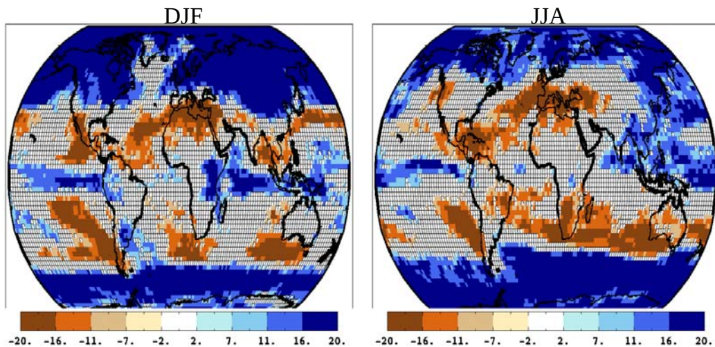
FIG. 3.1: Différence entre le nombre de modèles donnant une diminution de précipitations et le nombre de ceux donnant une augmentation. Vingt modèles utilisés dans le cadre du 4 ème rapport du GIEC sont considérés ici (soit la quasi-intégralité des modèles disponibles). On contraste les périodes 1970-2000 et 2070-2100 pour le scénario SRES A1B. Les points pour lesquels moins de 75% des modèles donnent le même signe (soit une différence de plus ou moins 10) sont blancs afin de faire ressortir les zones où une cohérence de signe existe. (gauche) hiver boréal ; (droite) été boréal.
