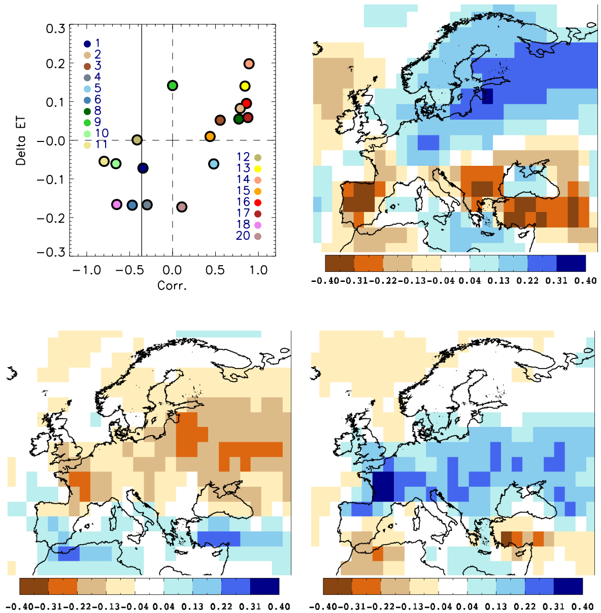
FIG. 10.21: (en haut à gauche) Changement d'évaporation moyenne sur la France entre les périodes 2080/2099 et 1961/1990 en fonction de la corrélation présente entre le total des flux radiatifs descendants en surface et l'évaporation en moyenne ( c_{re} ) sur la France. Le trait vertical plein indique la valeur de c_{re} pour SIM. (en haut à droite) Changements d'évaporation dans l'ensemble des modèles du GIEC. (en bas à gauche) Différence des changements d'évaporation entre le groupe A et l'ensemble des modèles. (en bas à droite) Différence des changements d'évaporation entre le groupe B et l'ensemble des modèles. Voir détails dans le texte.
