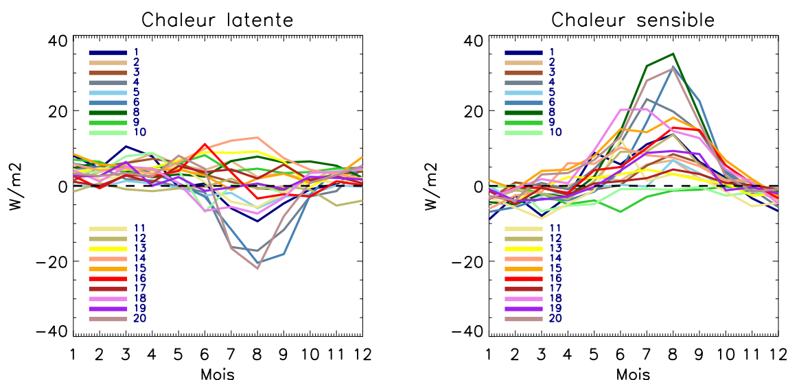
FIG. 10.19: Changement saisonnier entre les périodes 2080/2099 et 1961/1990 du flux de chaleur latente et du flux de chaleur sensible moyennés sur la France ( \text{W.m}^{-2} ). Les flux sont comptés positivement vers le haut, un changement positif correspond donc à une perte d'énergie pour la surface.
