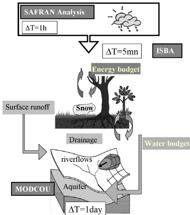
FIG. 4.1: Schéma récapitulatif du fonctionnement du système de modélisation hydrométéorologique SAFRAN-ISBA-MODCOU. Source : Habets et al., 2007 .
