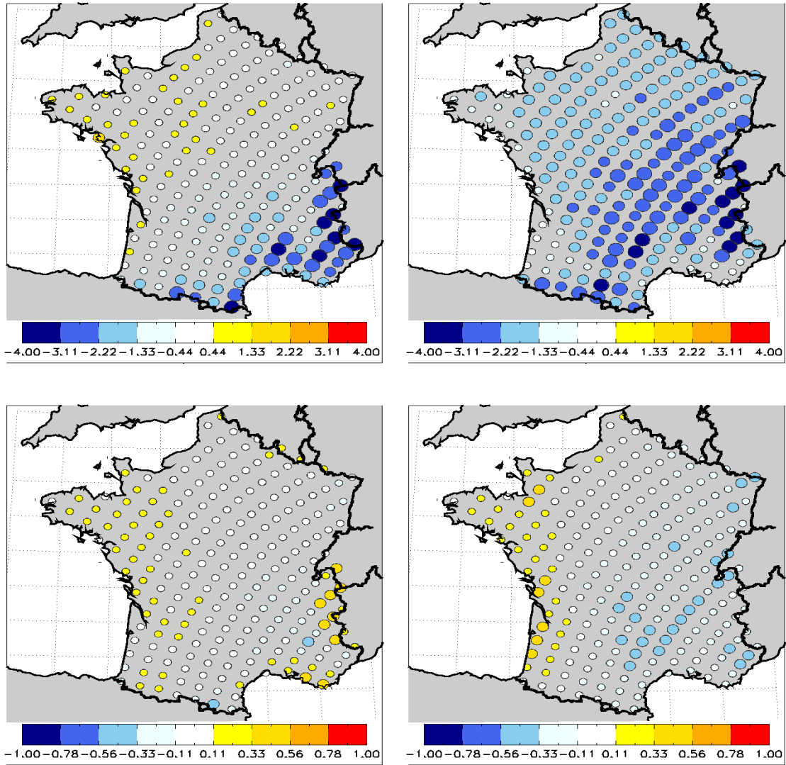
FIG. 7.4: Erreur sur la moyenne (MEAN en K, en haut) et la variance (VAR en K^2 , en bas) des températures ARPEGE-VR sur la période 1971-1999 par rapport à l'analyse SAFRAN, en hiver (à gauche) et en été (à droite)
