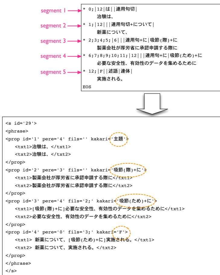
FIG. 11.9 – Exemple du résultat de la détermination du type de proposition
