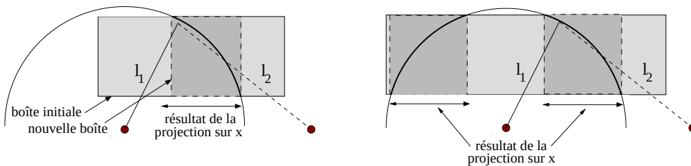
FIG. 1.4: Projection de la contrainte c_1 sur x .
