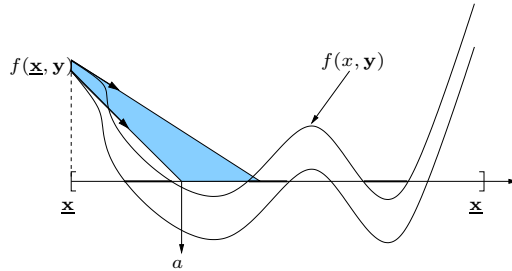
FIG. 6.8: Accélération du calcul de la box-cohérence. Le point a permet de séparer \mathbf{x} en deux sous-intervalles [\underline{x}, a] et [a, \overline{x}] , donc d'isoler l'un des continuums de solution.
