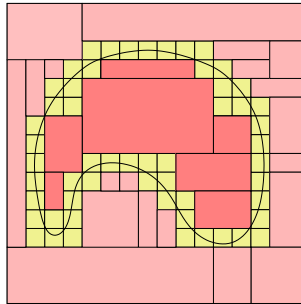
FIG. 2.8: Continuum et boîtes intérieures.
