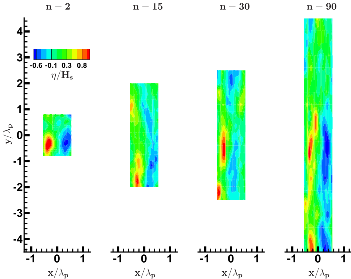
FIG. III.2.27 – Forme moyenne des vagues sclérates en fonction de la directionnalité
