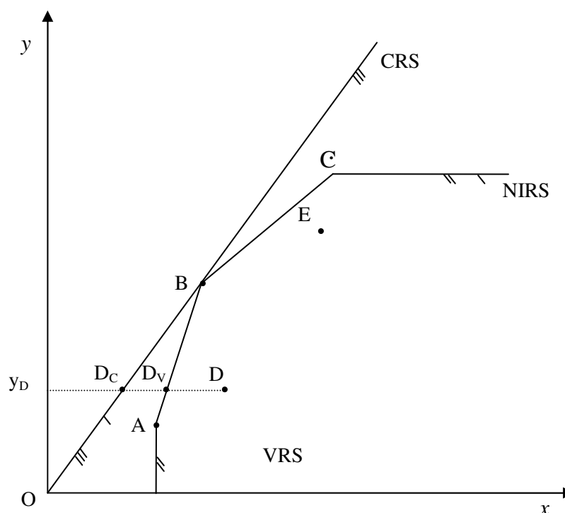
Figure 5.1. Mesure d'efficacité par la méthode de DEA
