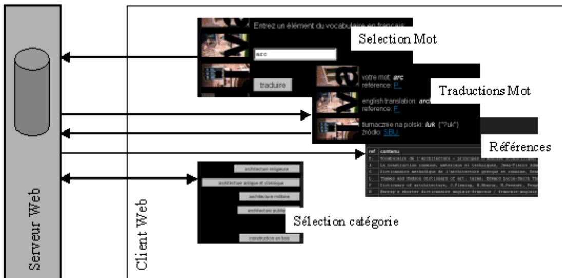
Figure 83 : Interface Web de l'outil DIVA
