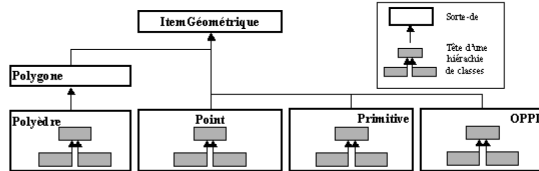
Figure 73 : Hiérarchie de concepts représentant les notions de géométrie utilisées dans l'implémentation JAVA
