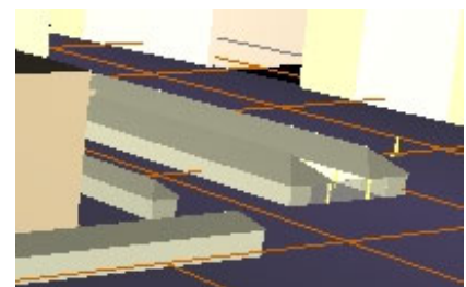
Figure 11 : Restitution des jarki olejne, powroźnicze, krupnicze, owsiane, śledziowe en VRML, incertitude sur la définition du portail symbolisée par un effet de transparence
