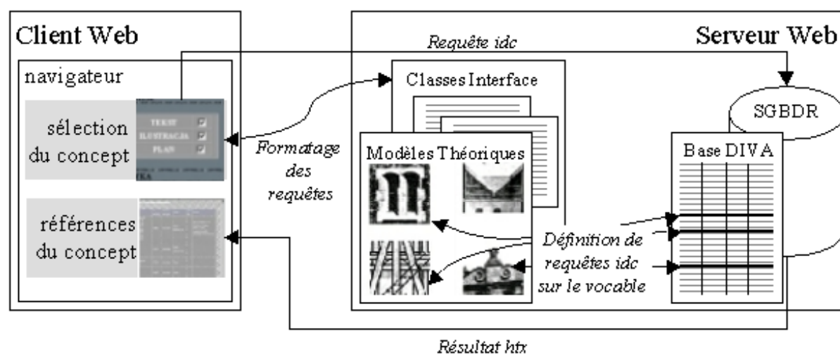
Figure 153 : Architecture Client-Serveur de l'application DIVA
