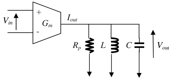
Fig. 3.1 Résonateur Gm-LC
