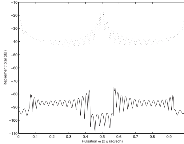
Fig. 4.8 Repliement total - méthode AGMC en bande passante et paramètres du tableau 4.1. En trait pointillé : \eta_S = 1, \eta_X = 0.98 . En trait plein : \eta_S = 0.86, \eta_X = 0.858 .
