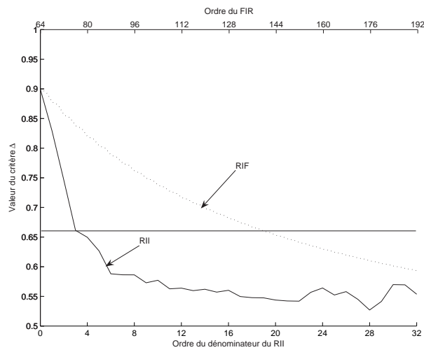
Fig. 4.14 Critère de qualité \Delta des BFH avec filtres de synthèse RII et RIF - synthèse ALMC à partir des paramètres du tableau 4.8
