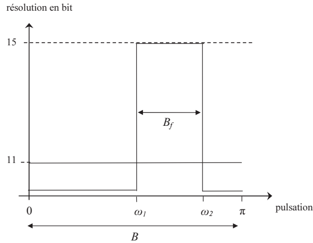
Fig. 4.13 Résolution avec et sans focalisation spectrale - paramètres du tableau 4.4.
