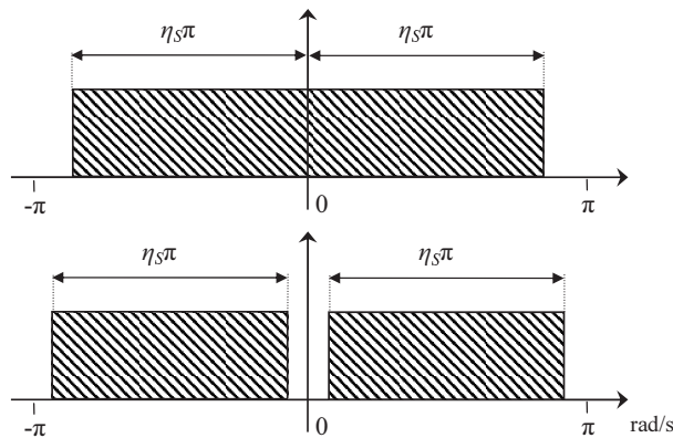
Fig. 4.6 Fréquences pour lesquelles on reconstruit le signal dans le cas d'un léger sur-échantillonnage. En haut : cas passe-bas, en bas : cas passe-bande
