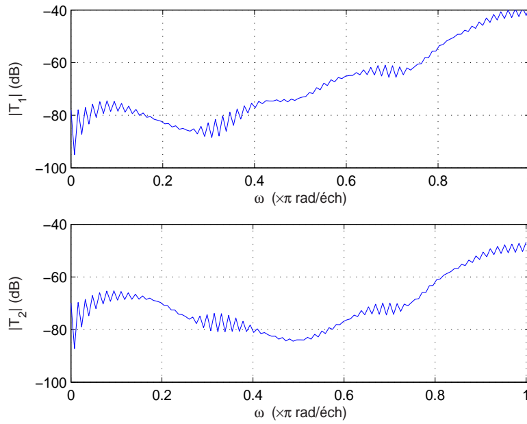
Fig. 3.9 Module des fonctions de repliement T_1(e^{j\omega}) et T_2(e^{j\omega}) - méthode TFI et paramètres du tableau 3.1
