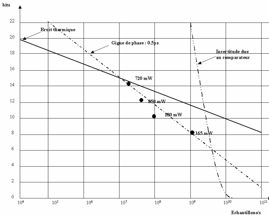
Fig. 2.3 Limitations de la résolution en fonction de la fréquence d'échantillonnage
