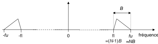
Fig. 4.2 Densité spectrale de puissance d'un signal continu en bande passante
