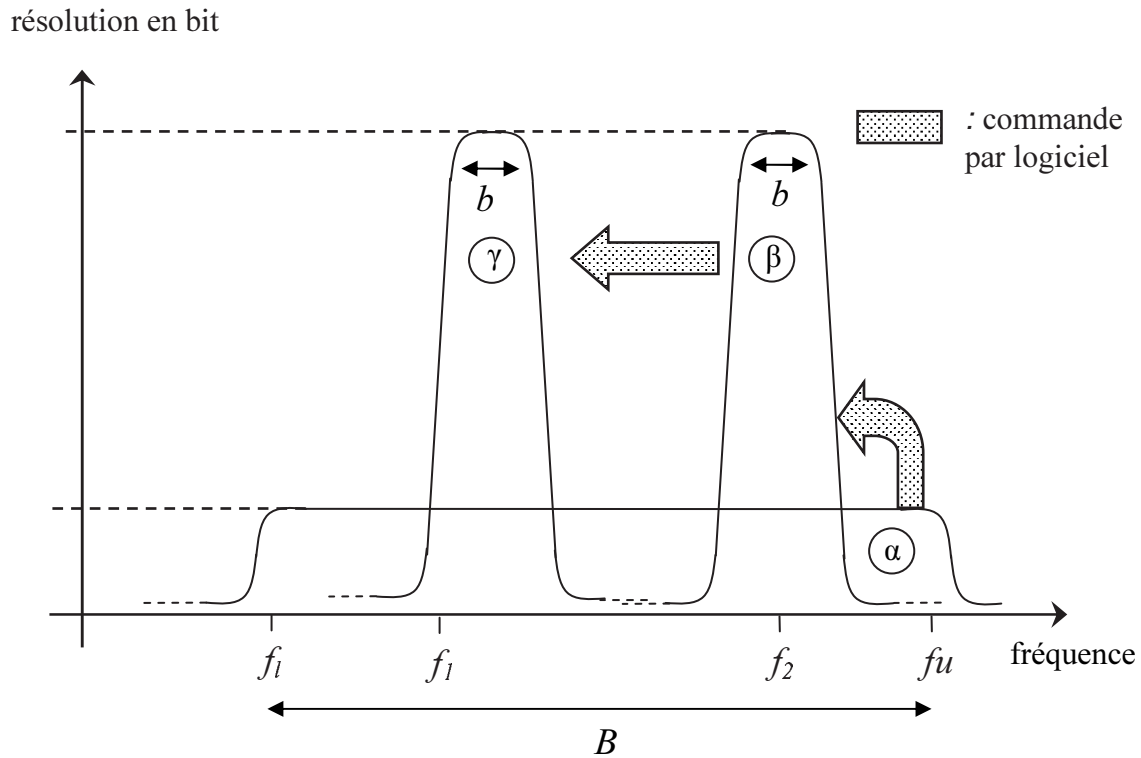
Fig. 2.5 Focalisation spectrale
