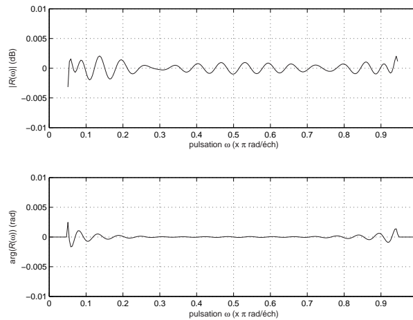
Fig. 4.9 Distorsion - méthode AGMC en bande passante - paramètres du tableau 4.4.
