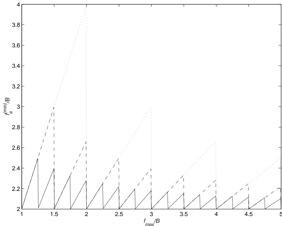
Fig. 4.1 Fréquence d'échantillonnage minimale ( f_e^{(min)} ) en fonction de la fréquence maximale ( f_{max} ) - en petits pointillés : pour un seul CAN; en gros pointillés : pour un BFH à quatre voies; en ligne pleine : pour un BFH à huit voies
