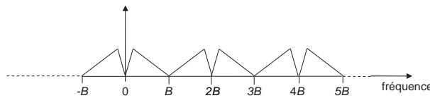
Fig. 4.3 Densité spectrale de puissance d'un signal en bande passante (cas N impair) échantillonné à 2B
