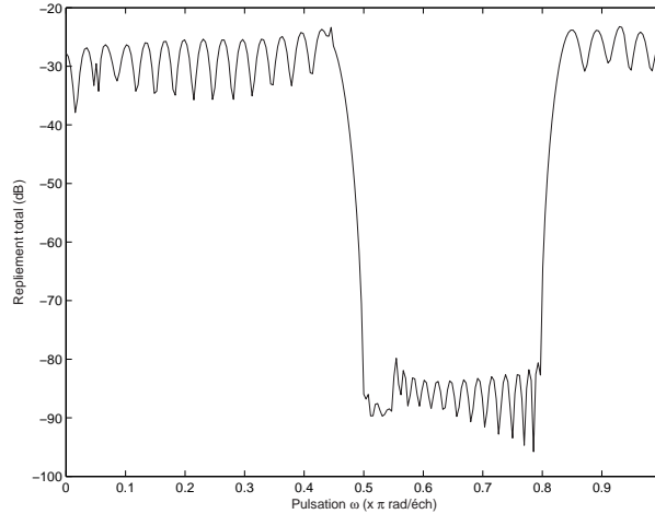
Fig. 4.12 Repliement total - méthode AGMC en bande passante avec focalisation spectrale - paramètres du tableau 4.4.
