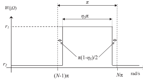
Fig. 4.5 Exemple de fenêtre de pondération
