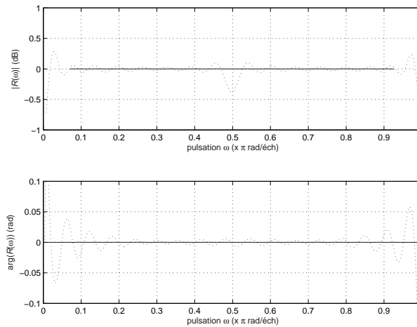
Fig. 4.7 Distorsion - méthode AGMC en bande passante - paramètres du tableau 4.1. En trait pointillé : \eta_S = 1, \eta_X = 0.98 . En trait plein : \eta_S = 0.86, \eta_X = 0.858 .
