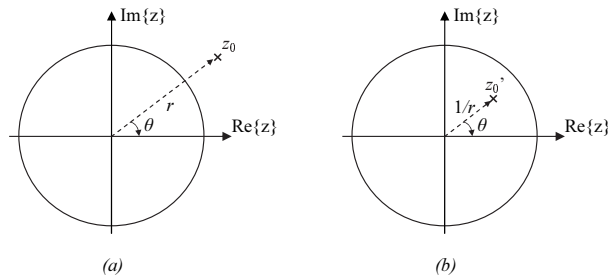
Fig. 4.15 (a) Pôle initial , en dehors du cercle unité. (b) pôle final, ramené dans le cercle unité après inversion du module
