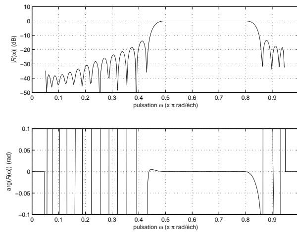
Fig. 4.11 Distorsion - méthode AGMC en bande passante avec focalisation spectrale - paramètres du tableau 4.4.
