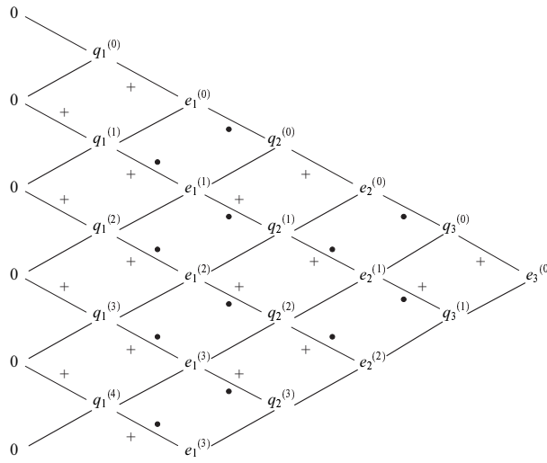
Fig. 4.16 Table « quotient-difference »
