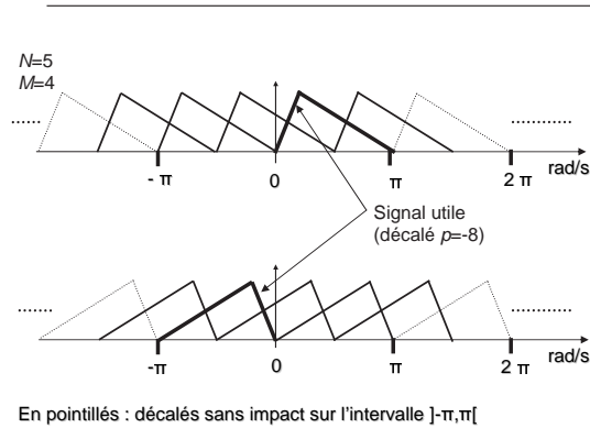
Fig. 4.4 Spectres décalés
