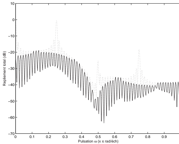
Fig. 3.15 Replieement total - méthode ALMC et paramètres du tableau 3.7. En trait pointillé : \eta_X = 1 . En trait plein : \eta_X = 0.9 .
