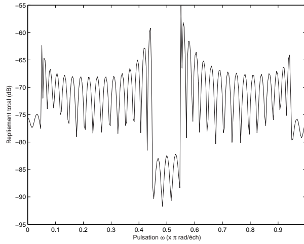
Fig. 4.10 Repliement total - méthode AGMC en bande passante - paramètres du tableau 4.4.
