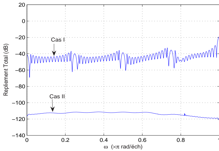
Fig. 3.20 Repliement total - méthode AGMC et paramètres du tableau 3.9.
