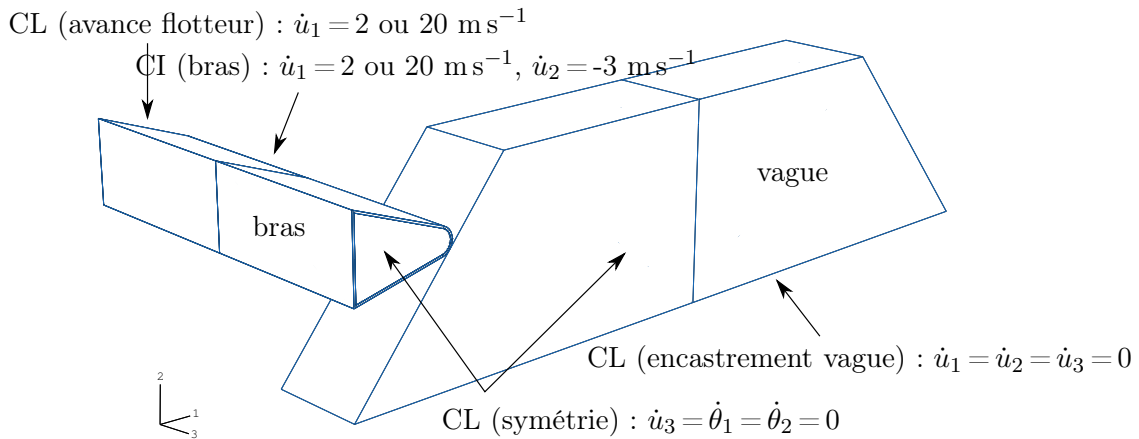
FIG. 5.10 – Chargements utilisés pour la modélisation des impacts hydrodynamiques
