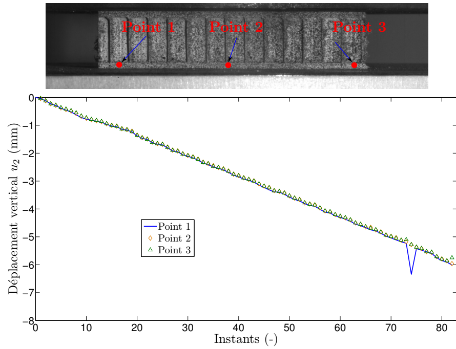
FIG. 3.21 – Comparaison des déplacements verticaux de trois points
