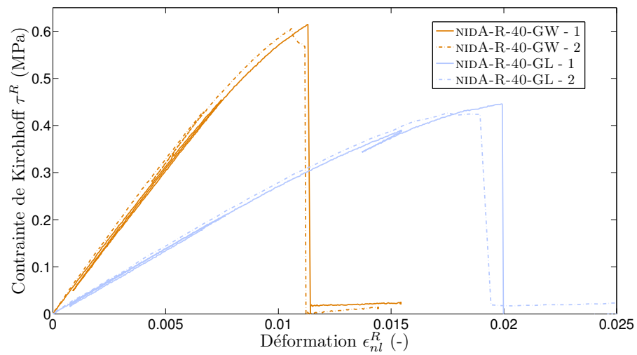
FIG. 3.20 – Réponses en cisaillement des NIDA-R-40
