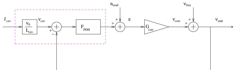
FIG. 6.2 – Schématisation du fonctionnement de l'asservissement, lorsque l'écart à résonance est plus petit que la largeur de raie de la cavité. La longueur de la cavité l_{cav} est une référence de fréquence \nu_{cav} , lorsque les perturbations considérées ont des fréquences plus petites que l'intervalle spectral libre. La fonction F_{PDH} traduit en un signal électrique l'écart à résonance. Dans le domaine fréquentiel, un facteur réel de sensibilité et un simple pôle, qui est le pôle de la cavité, représentent cette fonction de transfert, si les fréquences considérées sont très inférieures à l'intervalle spectral libre. L'ensemble entre traits hachurés représente le discriminateur Fabry-Perot, qui inclut les procédés de modulation/démodulation de la méthode Pound-Drever-Hall. L'écart mesuré \epsilon contient un bruit de lecture n_{read} . Le bloc G_{corr} représente l'électronique de correction et l'actionneur effectif. Le signal \nu_{corr} vient compenser le bruit propre du laser \nu_{free} , de sorte que le laser incident sur la cavité est maintenant stabilisé en fréquence.
