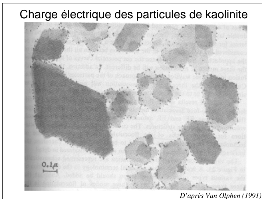
FIG. 3.3.7. Preuve expérimentale de la charge électrique des particules de kaolinite : les points adsorbés sur les surfaces latérales de la kaolinite sont des nanoparticules d'or (chargées négativement), y révélant ainsi l'existence d'une charge positive, extrait de [65].
