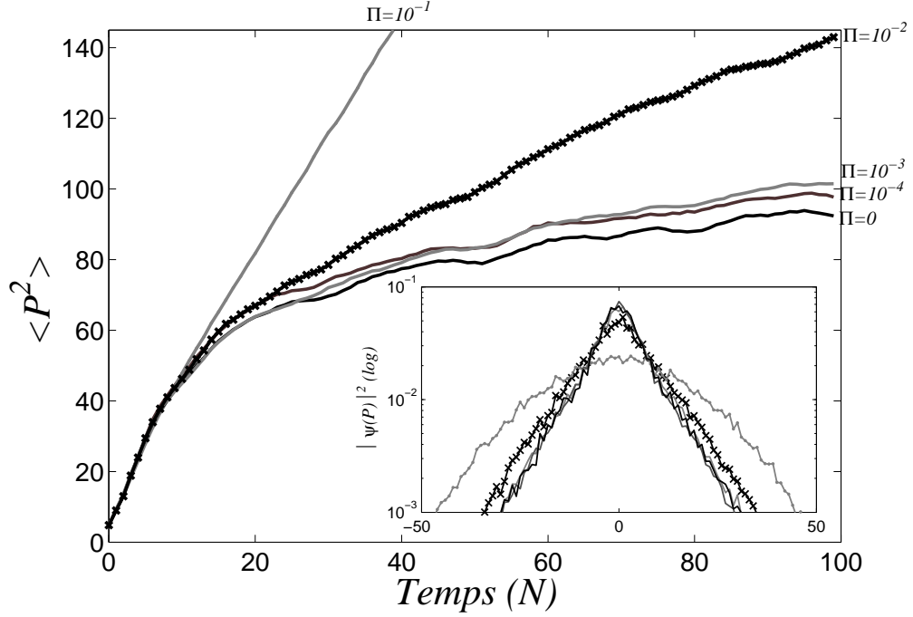
FIG. 2.23 – Évolution de l'énergie cinétique du kicked rotor (simulation numérique) pour K = 10 , \hbar k = 3, 46 et pour des probabilités d'émission spontanée par pulse ( \Pi ) de 0 , 10^{-4} , 10^{-3} , 10^{-2} et 10^{-1} . En encart, les distributions en impulsion correspondantes après 100 pulses. Tant que \Pi \lesssim 10^{-3} , la décohérence n'est pas suffisante pour altérer significativement le phénomène de localisation dynamique, la forme exponentielle est préservée et l'énergie cinétique tend à saturer. Si la probabilité d'émission spontanée par pulse est trop élevée ( \Pi > 10^{-3} ), la distribution en impulsion tend vers une forme gaussienne et un régime diffusif persiste.
