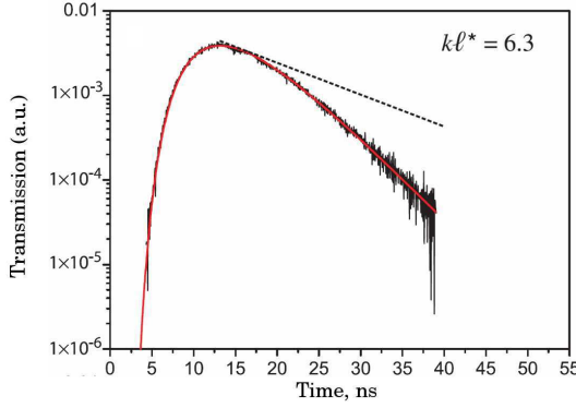
FIG. 3.11 – Coefficient de transmission dépendant du temps T(t) mesuré par M. Störzer et coll. [58] dans le régime diffusif ( k\ell > 1 ). Les données sont parfaitement décrites par l'Éq. (3.4) multipliée par \exp(-t/\tau_a) (ligne continue). La ligne pointillée montre \exp(-t/\tau_a) avec \tau_a qui résulte de la régression des données. Pour les temps longs, la décroissance de T(t) est exponentielle.
