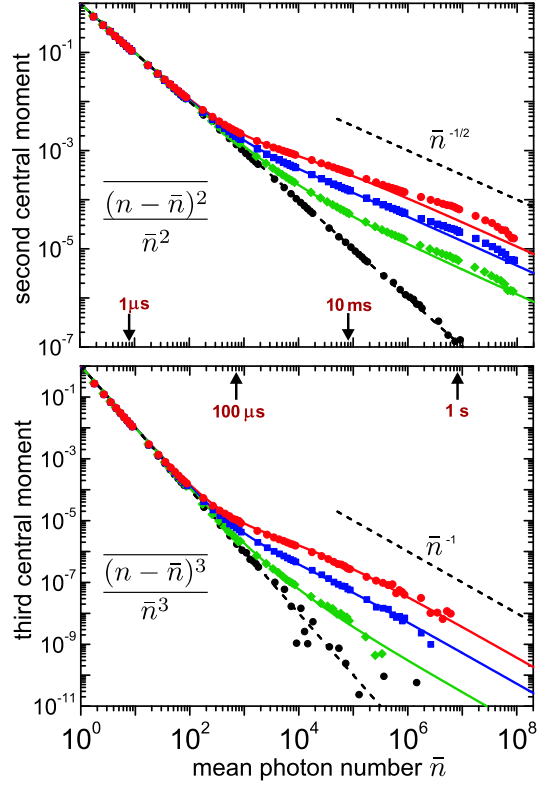
FIG. 4.4 – Deuxième (haut) et troisième (bas) moments centraux de la distribution de comptage de photons P(n, \bar{n}) . Les lignes correspondent à des tailles w différentes de la tache focale du faisceau laser, du bas vers le haut : faisceau collimaté ( w \rightarrow \infty ), w = 23,5 \mu\text{m} , 9,8 \mu\text{m} , et 3,4 \mu\text{m} . Les lignes pleines sont les résultats théoriques. Pour le faisceau collimaté, le deuxième et le troisième moments suivent les lois en 1/\bar{n} et 1/\bar{n}^2 (lignes pointillées) respectivement. Pour un faisceau focalisé, ils suivent les asymptotes 1/\bar{n}^{1/2} et 1/\bar{n} (lignes pointillées) pour \bar{n} \rightarrow \infty .
