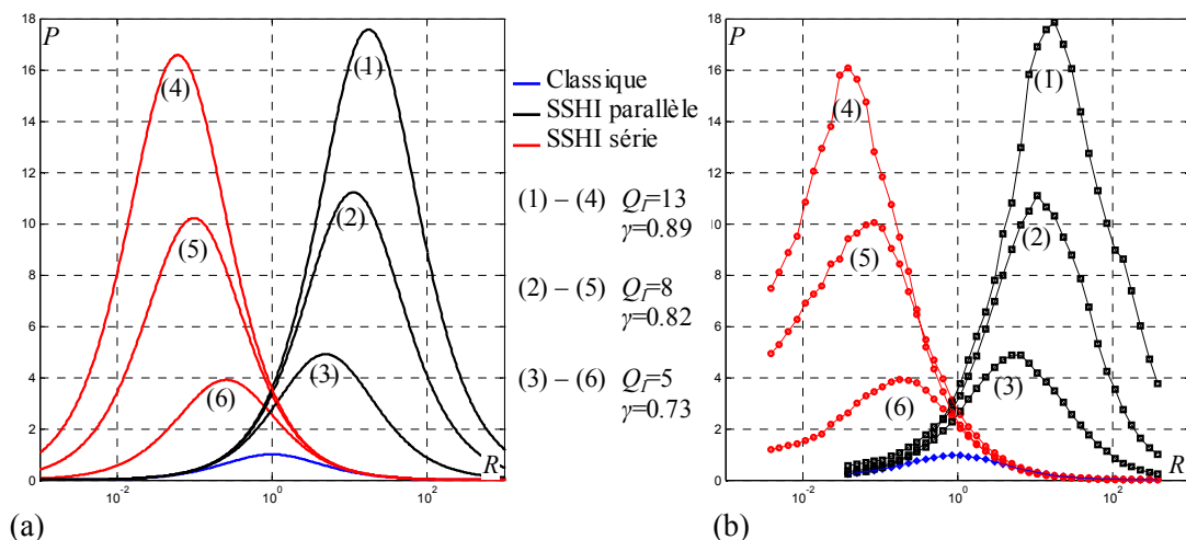
Figure 6-9 Puissances en fonction de la résistance de charge pour les techniques SSH séries et parallèles, pour différentes valeurs de \gamma : (a) résultats théoriques, (b) résultats expérimentaux.
