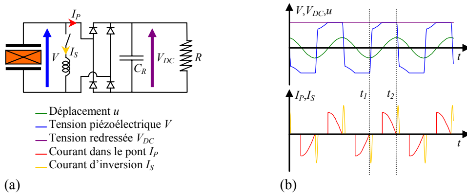
Figure 4-4 Technique SSHI continue : (a) dispositif, (b) formes d'ondes associées en régime sinusoïdal permanent
