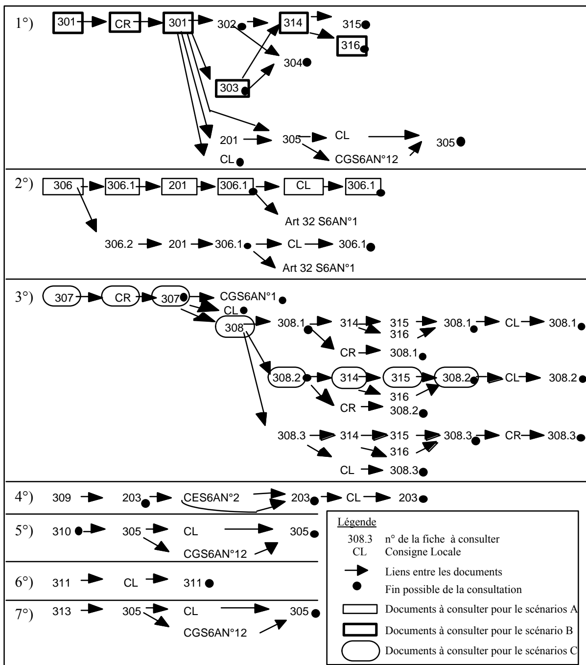
Figure 12 : Schéma simplifié des renvois entre les documents à l'usage des aiguilleurs
