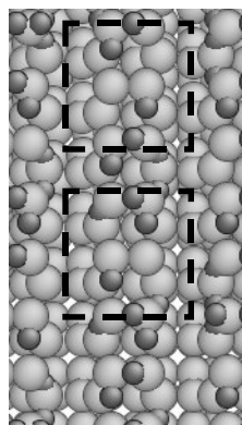
Figure IV. 23 : Deux défauts de type « liaison dimère non oxydée ». Les atomes d'oxygène sont en noir et les atomes de silicium sont en gris.
