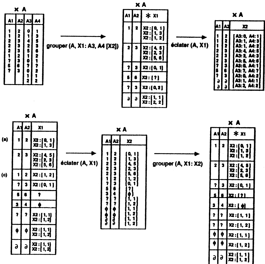
Figure 4.8 Enchaînement d'opérations grouper et éclater
