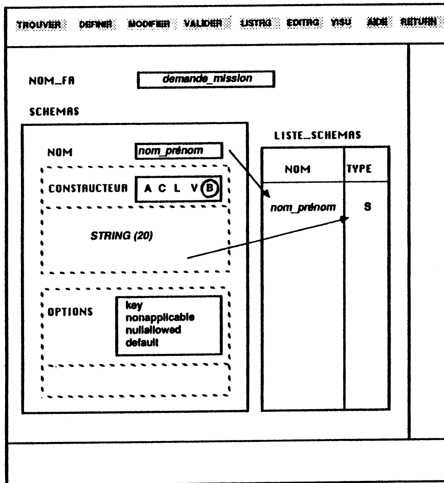
Figure 7.6 : Définition du FA demande_mission - élément nom_prénom
