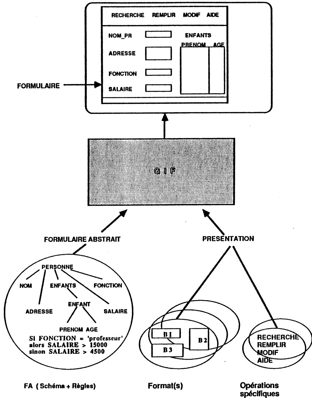
Figure 2.1 : Concepts du modèle de formulaires complexes
