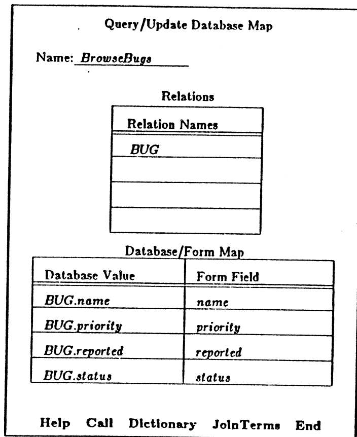
Figure 1.12 : Définition de l'association BugForm - BD
