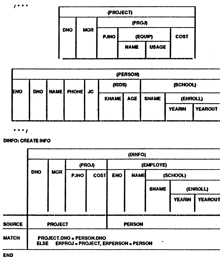
Figure 1.4 : Exemple de procédure OPAS
