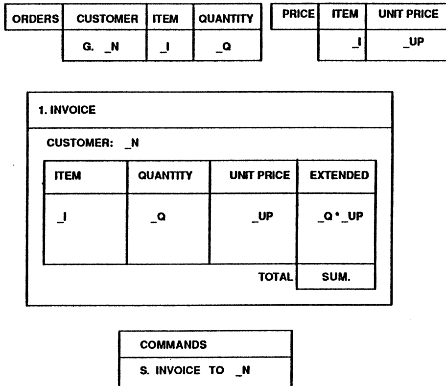
Figure 1.2 : exemple de programme pour produire une facture
