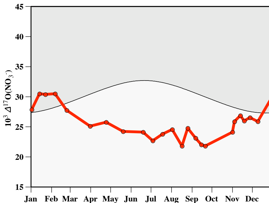
Figure 3.1 – Cycle saisonnier de \Delta^{17}\text{O}(\text{NO}_3^-) en Californie. La surface grisée représente les variations de la durée du jour (de 0 à 24h). D'après Michalski et al. (2003).
