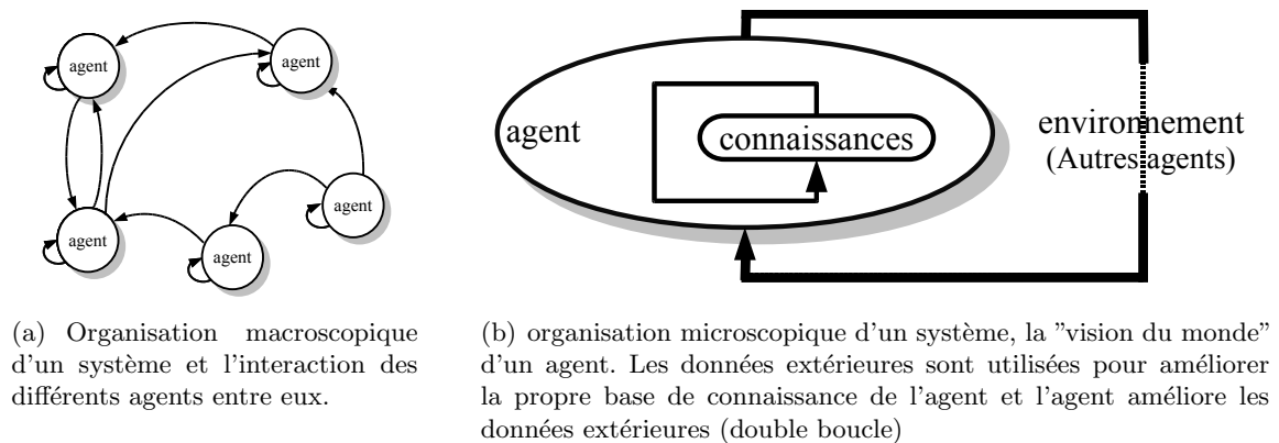
FIG. 5.11 – La double boucle des agents dans blexisma
