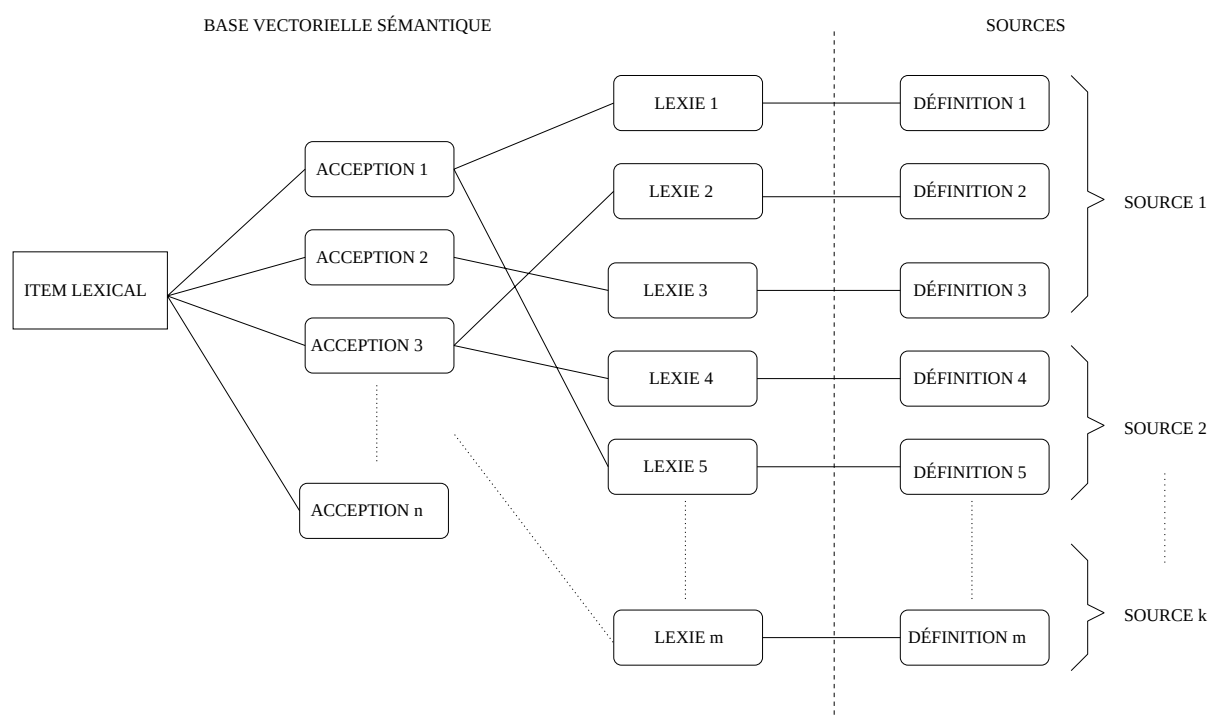
FIG. 5.4 – Organisation générale de la représentation du sens pour un item lexical.
