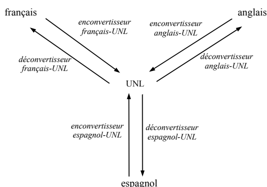
FIG. 6.1 – Principe d’UNL
