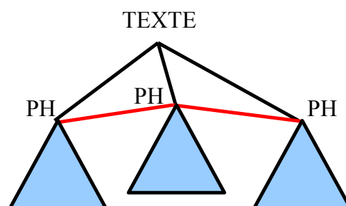
FIG. 7.8 – Liens interphrases.
