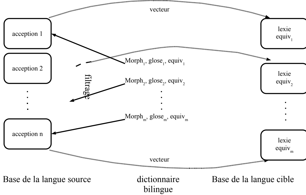
FIG. 8.3 – Le processus de mise en correspondance entre termes et acceptions cible et source
