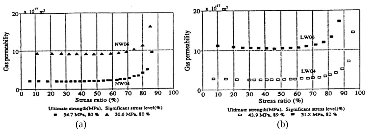
Figure 1.20 : Evolution de la perméabilité avec le taux de chargement pour (a) un béton à granulats normal et (b) un béton à granulats léger (d'après Sugiyama et al. , 1996).
