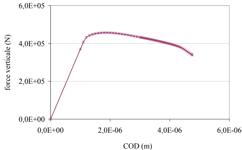
Figure 4.8 : Réponse globale du disque (D11) : force verticale – COD.
