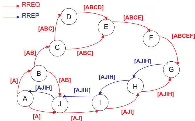
Figure 2.11 – Le principe de découverte de route dans le protocole DSR
