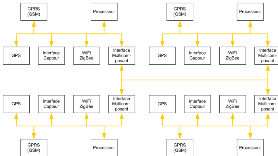
Figure 3.9 – Le principe d'un noeud e-CIVIC multisupport et tolérant aux pannes
