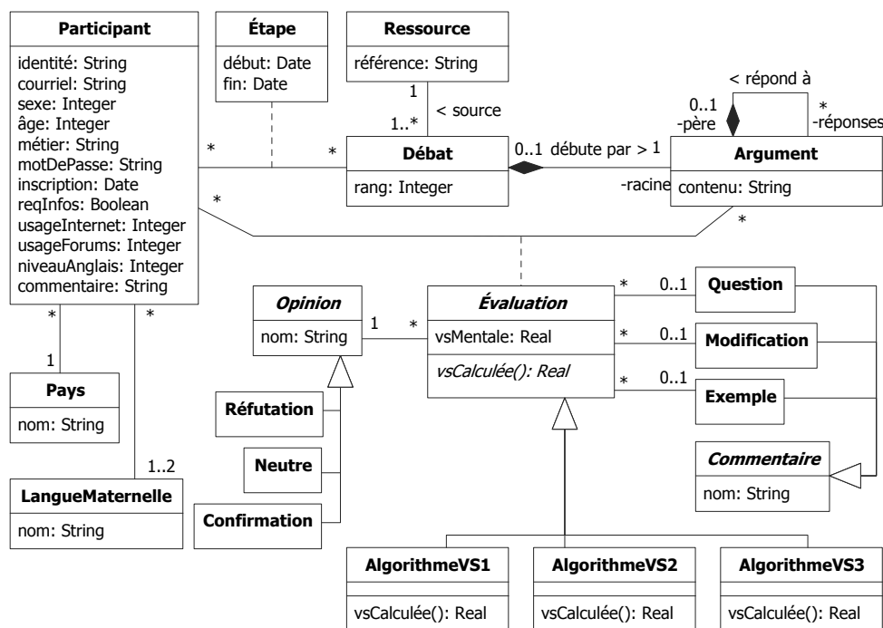
Figure III.2.3 – Diagramme des classes UML de la plate-forme d'expérimentation.
