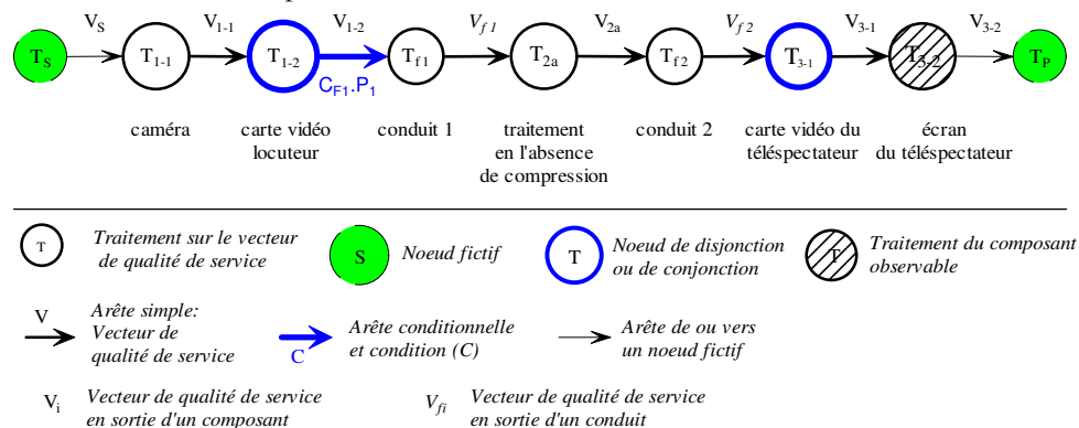
Figure 53: Exemple de Graphe d'évaluation de la qualité de service du Sous-Grouppe Image
