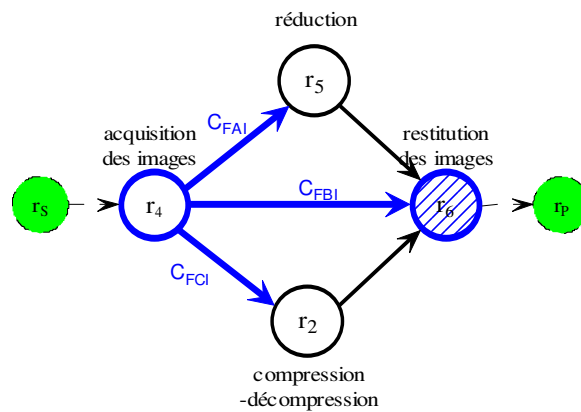
Figure 61 : Graphe des flots de contrôle du Sous-Groupe Image
