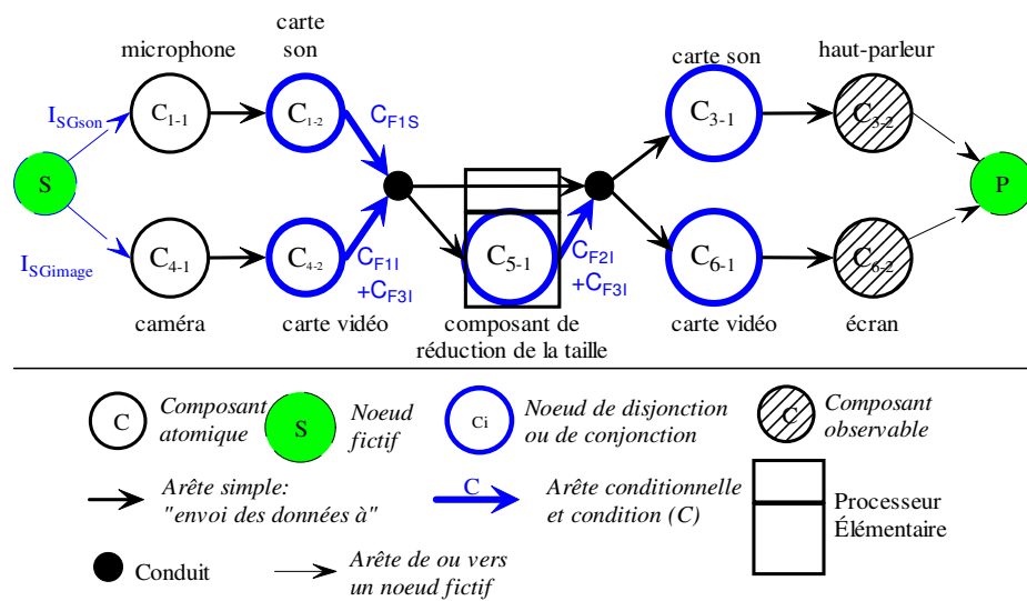
Figure 65 : Graphe d'une configuration du Groupe Téléspectateur
