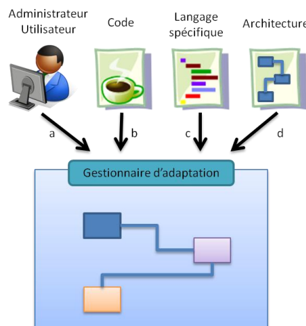
Figure 17. Gestionnaire d'adaptation et logique d'adaptation
