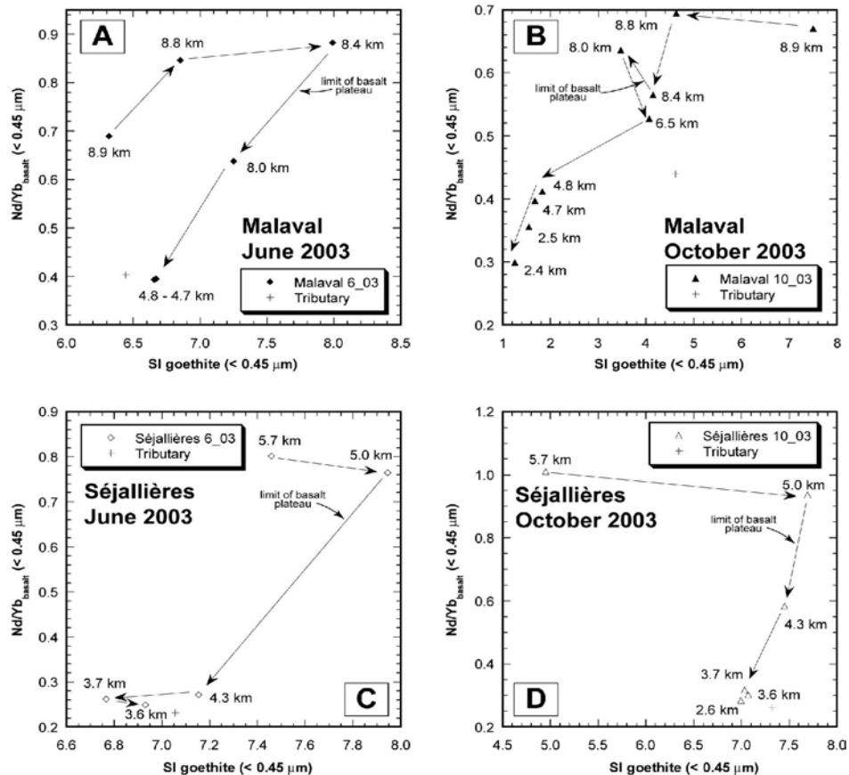
Fig. 48 : Variation de l'indice de saturation de la goethite et du rapport Nd/Yb de l'eau filtrée à 0.45 μm des ruisseaux Malaval et Séjallières avec la distance. On constate pour les 2 paramètres une diminution des valeurs à partir du moment où le ruisseau a franchi le rebord du plateau basaltique (Fig. 7 de Steinmann et Stille, 2008).
