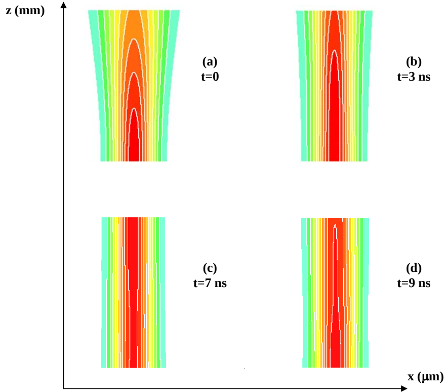
FIG. 3.7 – Calcul numérique de la propagation d'une impulsion laser de 10\text{ ns} dans un cristal BTO de longueur 6\text{ mm} à différents instants (a) t = 0 (b) t = 3\text{ ns} (c) t = 7\text{ ns} (d) t = 9\text{ ns} .
