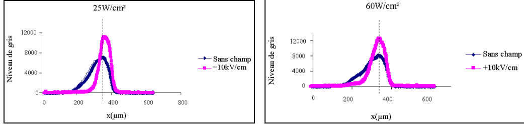
FIG. 4.11 – Mesure de l’auto-déviaton du faisceau pour w = 25 \mu\text{m} , \lambda = 1.56 \mu\text{m} à (a) I = 25 \text{ W/cm}^2 (b) I = 60 \text{ W/cm}^2 . Le trait en pointillé indique la position de l’intensité maximale du faisceau sans champ appliqué.
