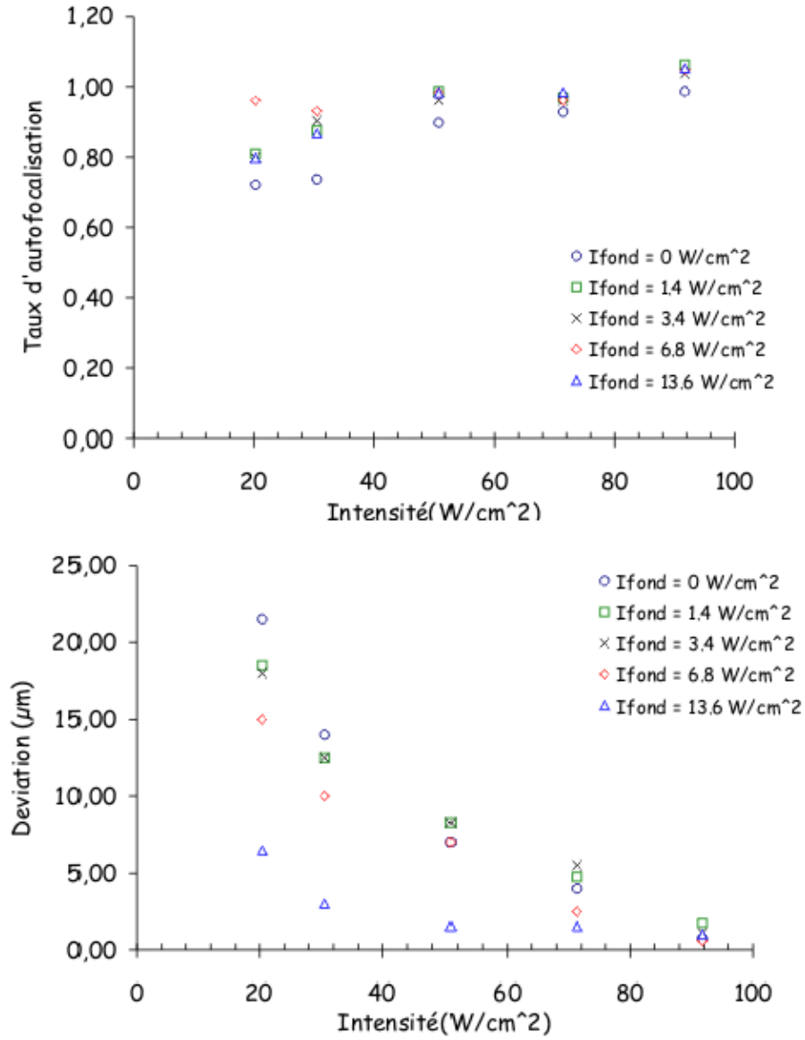
FIG. 4.14 – Evolution du taux d'autofocalisation et de la déviation du faisceau en fonction de l'intensité du faisceau et de l'intensité d'éclairage de fond pour une température de 293\text{ K} . Longueur d'onde du faisceau \lambda = 1.56\text{ }\mu\text{m} , longueur d'onde d'éclairage de fond \lambda = 1.06\text{ }\mu\text{m}
