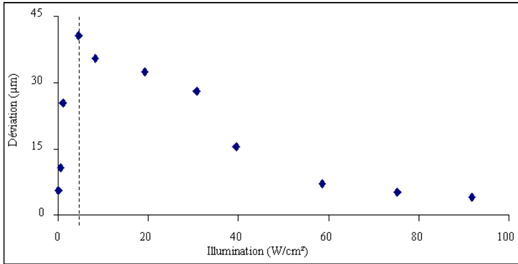
FIG. 4.12 – Auto-déviaton du faisceau en fonction de l’intensité pour w = 25 \mu\text{m} et \lambda = 1.56 \mu\text{m} . Le trait en pointillé indique le niveau de l’intensité du faisceau où la déviation est maximale.
