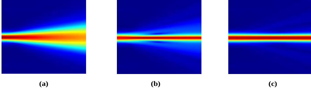
FIG. 3.6 – Simulations numériques de la formation du soliton spatial stationnaire pour r = 10 , N = 1 et D = 0 à différents instants : (a) t = 0 ; (b) t = T_e/5 ; (c) t = T_e .
