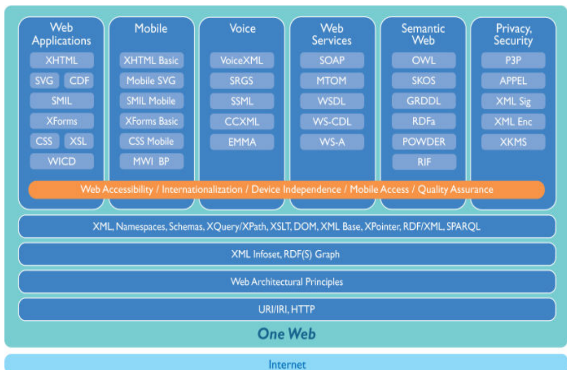
Figure 26. Piles des activités de standardisation au W3C reposant sur les structures d'arbre de XML et de graphe de RDF (source : www.w3.org ).
