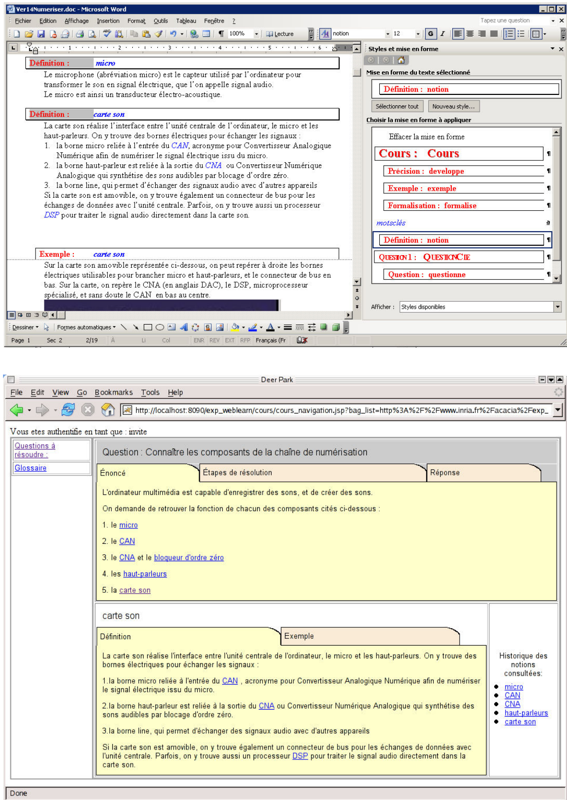
Figure 12. Cours entré sous Microsoft Word (en haut) en utilisant des styles prédéfinis et (en bas) le même cours automatiquement réorganisé pour des séances de TP ou TD
