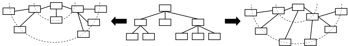
Figure 100. Méthodes ascendantes et descendantes d'attribution d'un angle à une classe de l'ontologie
