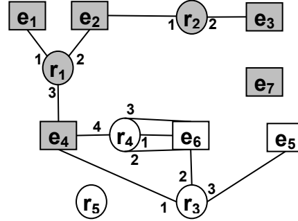
Figure 47. Sous-ERGraph induit par E_{G'} = \{e_1, e_2, e_3, e_4, e_5, e_6, e_7\}
