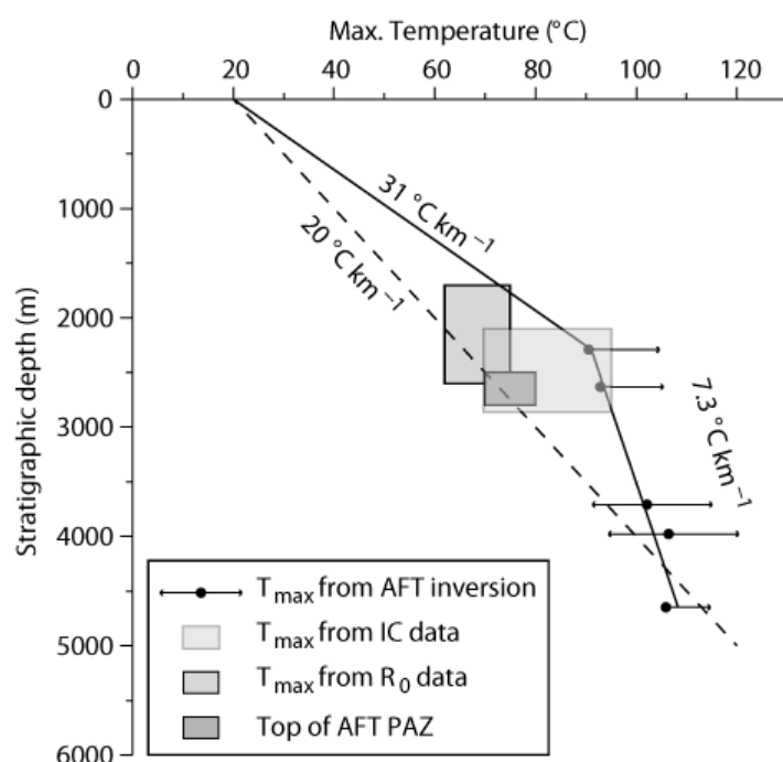
FIG. 5.6 – Paléotempératures maximales atteintes par les échantillons partiellement recuits prédites par les inversions d'AFTsolve en fonction de la profondeur stratigraphique. Les points représentés correspondent au meilleur modèle lié à chaque échantillon, et la barre d'erreur au maximum et au minimum autorisé pour les modèles acceptables. Pour comparaison, le champ de paléotempératures maximales issu des valeurs de réflectance de la vitrinite ( R_0 ; L. Martinez, communication personnelle, 2003) et de cristallinité de l'illite (IC; Huyghe et al. (2005)) est respectivement représenté; d'après van der Beek et al. (2006).
