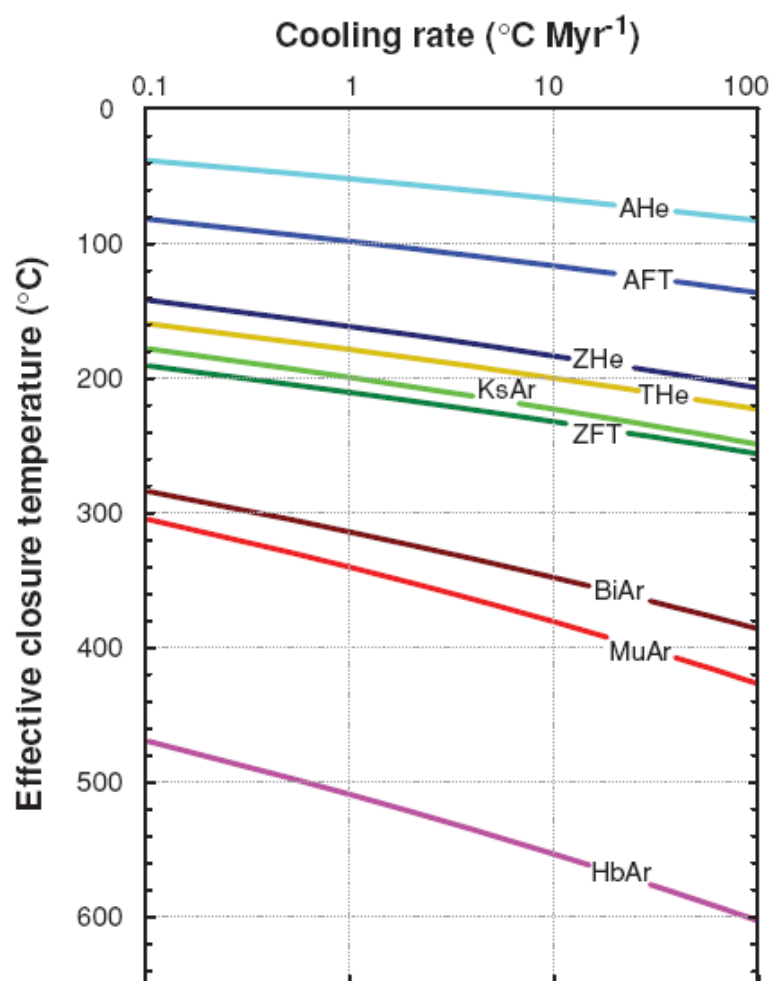
FIG. 2.2 – Estimation de la température de fermeture effective en fonction du taux de refroidissement pour les thermochronomètres He, FT et Ar (Reiners et Brandon 2006).
