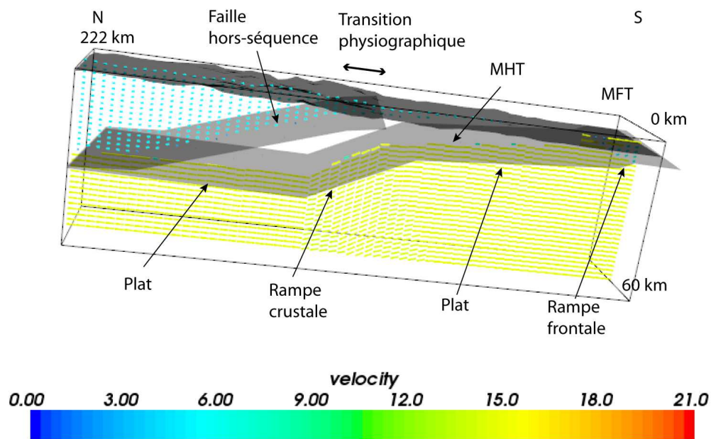
FIG. 3.1 – Géométrie de failles (MFT, MHT et hors séquence) implémenté dans la modélisation, et champ de vitesses associées (en \text{km}.\text{My}^{-1} ). Ici, la pente de la rampe du MHT est de 17.8^\circ .
