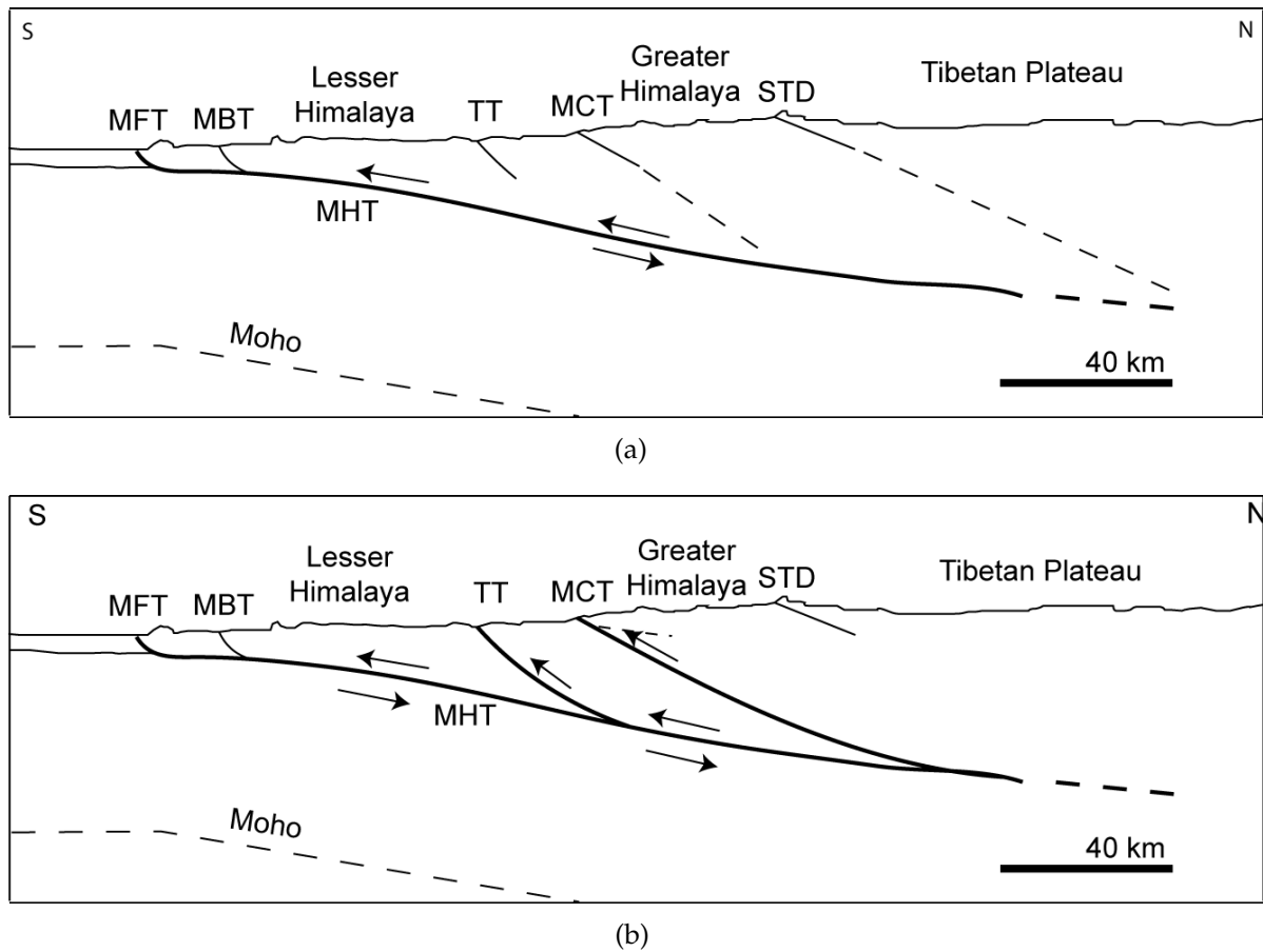
FIG. 1.16 – Modèles de déformation du front de la chaîne himalayenne. a) Modèle de Lavé et Avouac (2001) : la déformation est principalement accommodée au front de la chaîne grâce au MHT - MFT. b) Modèle de Hodges et al. (2004) : la déformation est accommodée à la fois au front de la chaîne par le couple MHT - MFT, mais aussi grâce à une réactivation hors séquence au niveau du front topographique. (Schémas modifiés d'après Hodges et al. (2004) ).
