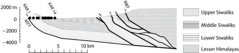
FIG. 5.2 – Coupe équilibrée de la Karnali River montrant la localisation des échantillons et la relation avec la structure tectonique locale ; modifié d'après Mugnier et al. (1999) , van der Beek et al. (2006) .
