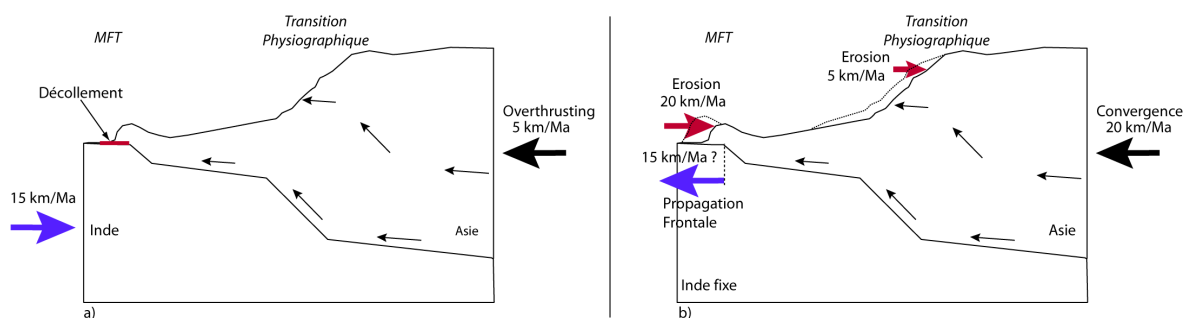
FIG. 5.10 – Schéma conceptuel donnant deux explications indépendantes expliquant le différentiel de vitesses observé entre la transition topographique et la zone du MFT. a) Décrolement du front des Siwaliks sur l'Inde ; b) Interprétation de la vitesse d'overthrusting en terme d'érosion différentielle, dans un repère fixé sur l'Inde.
