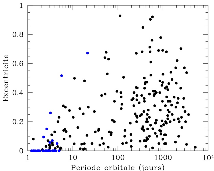
FIG. 1.5 – Diagramme Excentricité-Période orbitale des planètes connues. De la même manière que précédemment, les points noirs représentent les planètes dont la masse est minimale et les points bleus les planètes dont la masse est exacte.
