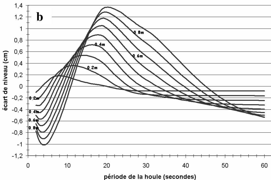
Fig. 6.13. – Effet de la houle sur le niveau moyen à l’intérieur du puits de tranquillisation. a. construit après la seconde guerre mondiale à Brest (d’après la figure C.6B de Simon (2007)) ; b. construit sous l’ère Chazallon et fonctionnant jusqu’en 1944. Chaque courbe représente, pour une amplitude de houle déterminée, la variation du niveau moyen (en cm) dans le puits en fonction de la période du signal externe.
