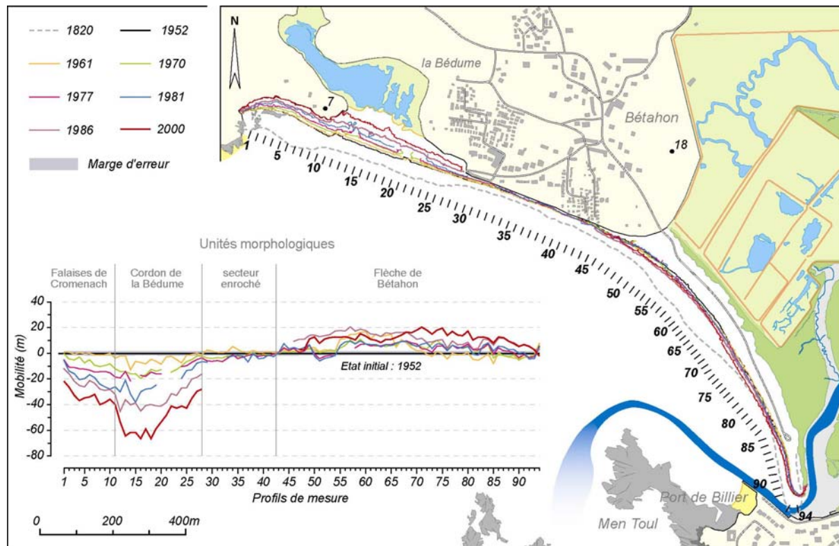
Figure 176 : Evolution des différentes unités morphologiques qui composent l'Anse de Bétahon entre 1820 et 2000.
