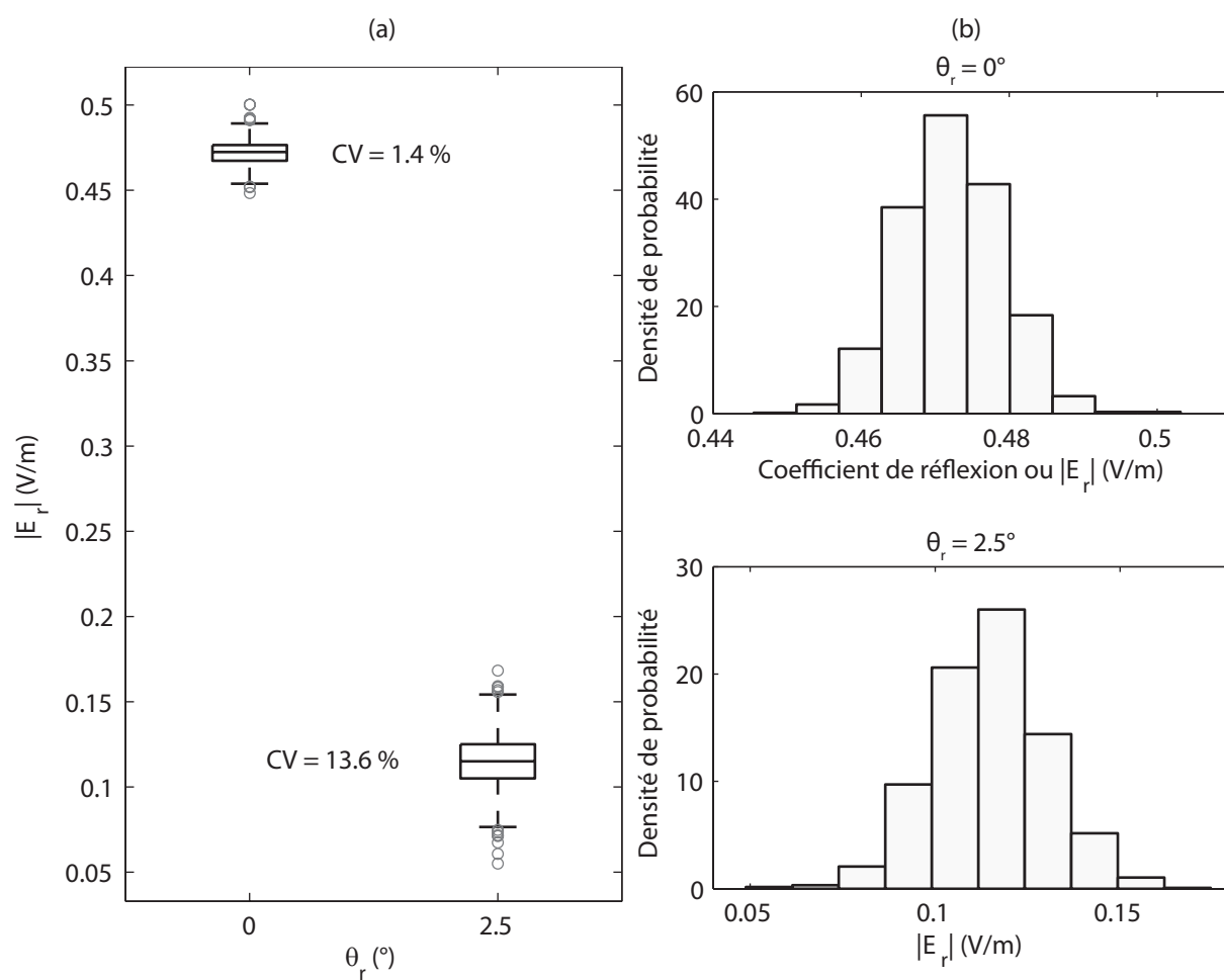
FIG. 4.18 – Résultats de l'étude statistique sur la distribution des fenêtres de dimensions 1\text{ m} \times 1\text{ m} pour une onde plane en incidence normale (a) Boxplots présentant la variation du champ réfléchi dans les directions spéculaire et non-spéculaire (b) Densités de probabilité du champ réfléchi dans les directions spéculaire et non-spéculaire
