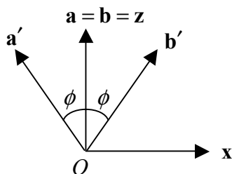
Figure B.1 Choix particulier des directions \mathbf{a} , \mathbf{a}' , \mathbf{b} et \mathbf{b}'
