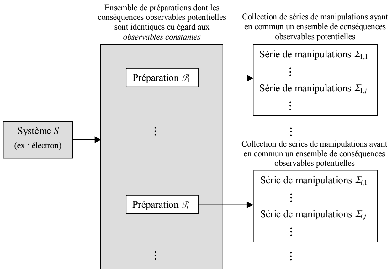
Figure 5.2 Lien entre un système S , un ensemble \{\mathcal{P}_i\} de préparations et un ensemble \{\{\Sigma_{1,j}\}, \dots, \{\Sigma_{i,j}\}, \dots\} de collections de séries de manipulations
