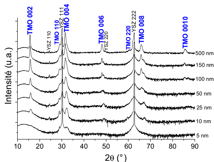
Figure 3.31 : diagrammes de diffraction \theta/2\theta de films de \text{TbMnO}_3 de différentes épaisseurs, déposés à 850^\circ\text{C} , avec \text{Tb/Mn} en solution = 1.2. Les intensités sont en échelle logarithmique.
