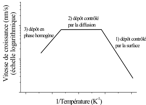
Figure 2.2 : représentation des différents régimes de croissance d'un film déposé par CVD en fonction de l'inverse de la température.
