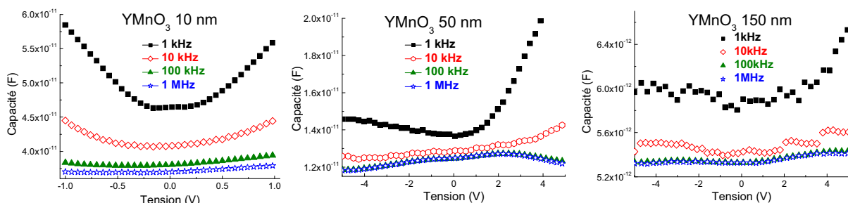
Figure 4.31 : mesures C(V) de films d' \text{YMnO}_3 de 10, 50 et 150 nm d'épaisseur déposés sur Pt/Si à 800^\circ\text{C} , sur des électrodes de 70 \times 70 \mu\text{m}^2 , à différentes fréquences.
