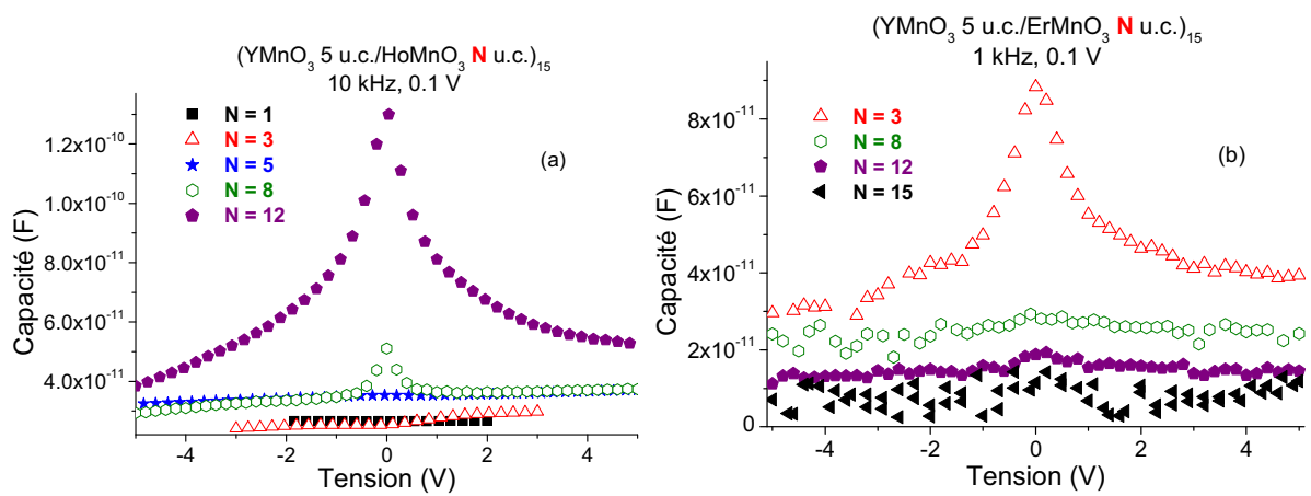
Figure 5.20 : mesures C(V) (a) de multicouches (YMnO 3 5 u.c./HoMnO 3 N u.c.) 15 déposées sur Pt/Si à 825°C et (b) de multicouches (YMnO 3 5 u.c./ErMnO 3 N u.c.) 15 déposées sur Pt/Si à 850°C - mesures effectuées sur des électrodes de surfaces 150x150 μm 2 .
