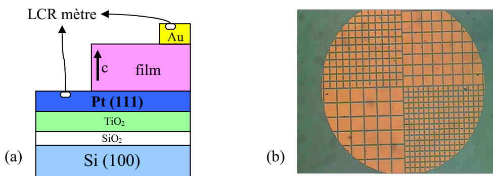
Figure 4.27 : (a) structure capacitive utilisée pour les mesures électriques - (b) image au microscope optique des électrodes d'or évaporées à travers un masque de carrés de 50x50, 70x70, 110x110 et 150x150 μm 2 .
