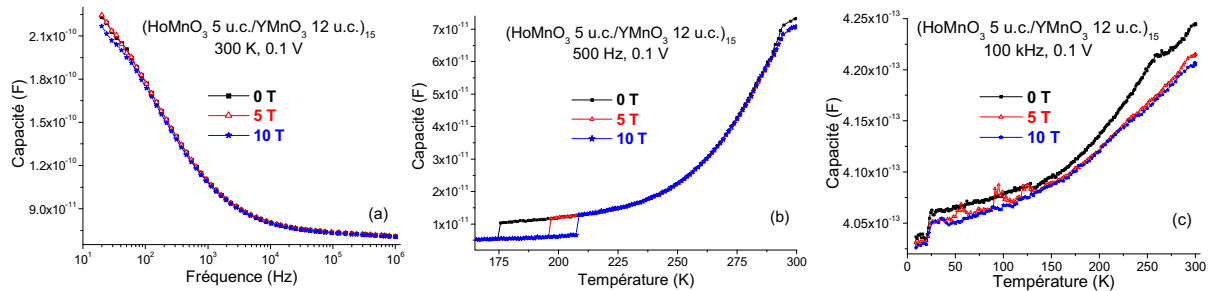
Figure 5.22 : différentes mesures de capacité en fonction de la température et de la fréquence et sous différents champs magnétiques d'une multicouche (HoMnO 3 5 u.c./YMnO 3 12 u.c.) 15 élaborée sur Pt/Si à 825°C - mesures effectuées sur des électrodes de surfaces 110x110 μm 2 , avec H/c.
