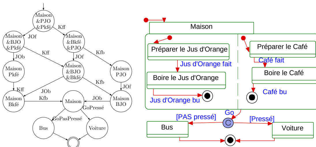
(a) diagramme d'état transition
