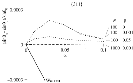
Fig. IV.74 : Evolution du déplacement du pic de diffraction (311) en fonction de la probabilité de fautes d'empilement \alpha . Le paramètre N correspond au nombre de plans (111) dans la colonne suivant la direction définie par le vecteur de diffraction \vec{S} . \beta est la densité de joint de macle (Velterop et al. , 2000)
