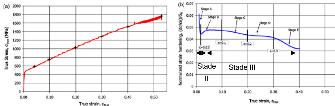
Fig. I.21 : Essai de traction en contrainte vraie en fonction de la déformation vraie (a) et durcissement normalisé en fonction de la déformation vraie pour un acier Fe22Mn0.6C avec une EFE de 18\text{mJ.m}^{-2} à température ambiante (Barbier et al. , Püschl, 2002)
