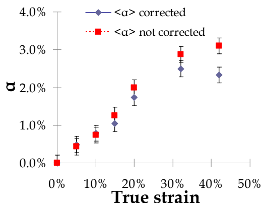
Fig. IV.107 : Evolution de la densité apparente moyenne de fautes d'empilement \langle \alpha \rangle avec la déformation vraie pour la nuance CC3 déformée en traction uniaxiale à température ambiante. Les mesures non corrigées sont le résultat de la moyenne des trois premiers pics (111), (200) et (220). Les mesures corrigées de \langle \alpha \rangle sont réalisées sur les pics (111), (200) et (220) et corrigées avec leur harmonique supérieur
