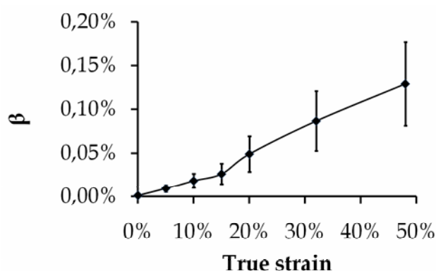
Fig. IV.108 : Evolution de la densité moyenne de fautes d'empilement \langle \beta \rangle avec la déformation vraie pour la nuance CC3 calculée à partir de la densité de faute apparente 1.5\alpha + \beta . L'incertitude est estimée directement à partir de l'écart-type des valeurs sur les onze pics de diffraction
