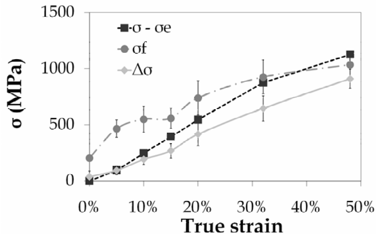
Fig. V.123 : Durcissement expérimental lors d'un essai de traction comparé aux durcissements calculés à partir des densités de dislocations ( \sigma_f ) et aux mesures de back-stress ( \Delta\sigma ) par diffraction à partir de A_L^B pour la nuance FeMn1000
