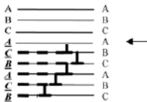
Fig. I.24 : Représentation schématisée du réarrangement des plans compacts autour d'une macle mécanique créée par le déplacement de dislocations partielles intrinsèques tous les plans atomiques. La flèche indique la position du joint de macle, plan miroir pour le réseau CFC (ALLAIN, 2004)
