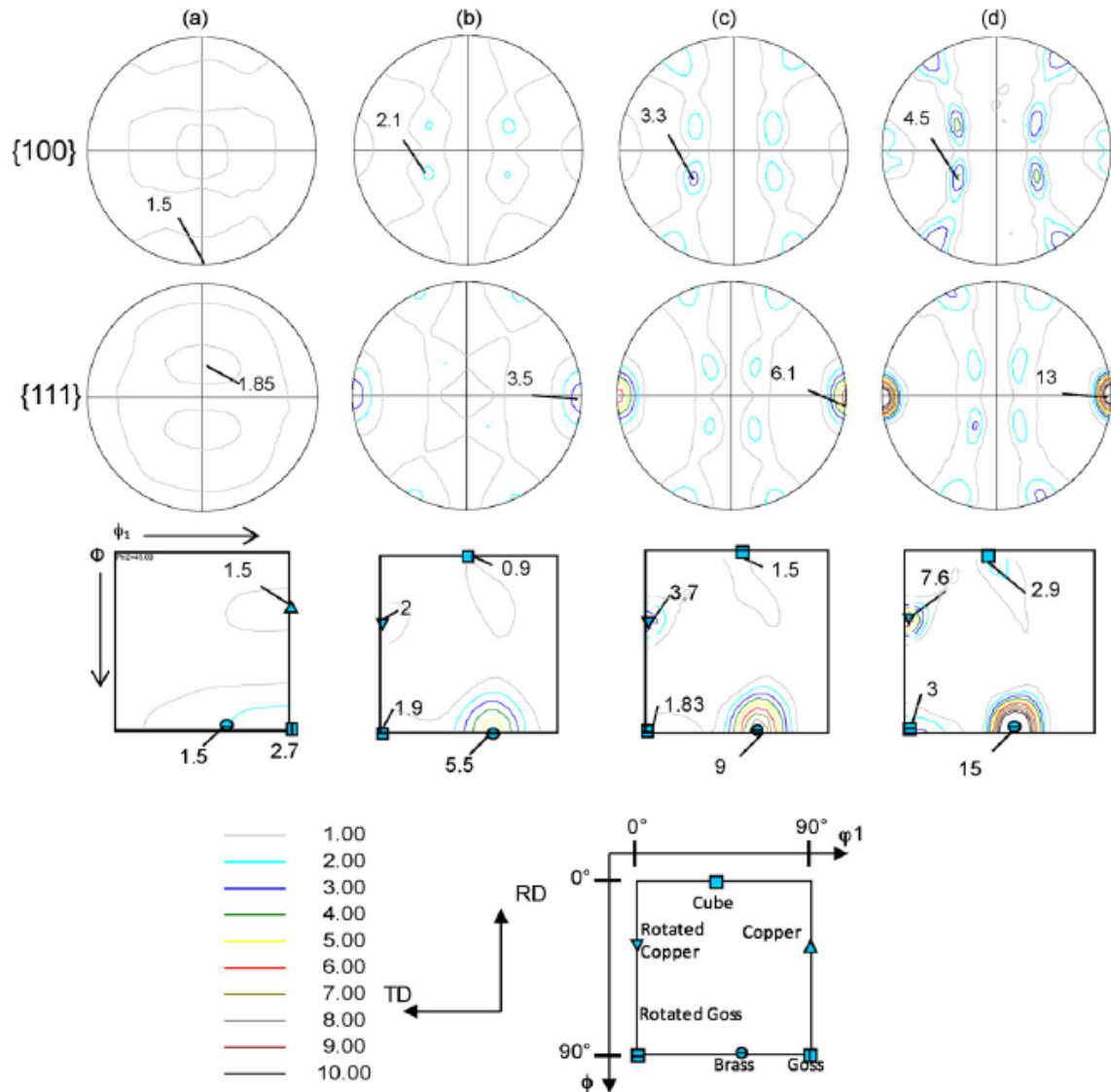
Fig. V.125 : Figures de pôle {100} et {111} mesurée en réflexion sur un diffractomètre de laboratoire avec un tube au cuivre sur une nuance Fe22Mn0.6C issue d'une coulée industrielle pour différents niveaux de déformation vraie (Barbier et al. , 2009). De gauche à droite 0%, 20%, 30% et 55% de déformation vraie
