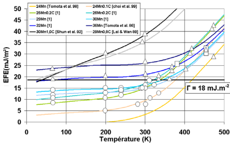
Fig. I.13 : Modélisation de l'EFE en fonction de la température pour des compositions correspondant aux alliages étudiés par différents auteurs (Remy & Pineau, 1976, Li & Hsu, 1997, Tomota et al. , 1986, Shun et al. , 1992, Tomota et al. , 1998, Choi et al. , 1999, Chen et al. , 1999). Les différents symboles représentant les mécanismes de déformation observés par les auteurs ont été reportés le long des courbes. ( \square : glissement seul, \Delta : maclage mécanique + glissement, \circ : transformation martensitique \varepsilon + glissement) (ALLAIN, 2004). La référence notée [1] correspond à (Remy & Pineau, 1976)
