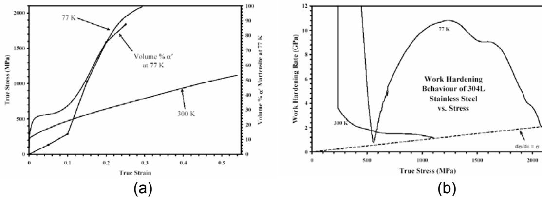
Fig. I.30 : Essai de traction (a) pour un acier inoxydable 304L à température ambiante et 77K et le taux d'écrouissage associé en fonction de la contrainte (b). La ligne pointillée sur (b) correspond au critère de Considère. La déformation à 77K met en évidence un très fort effet TRIP (Spencer et al. , 2004)
