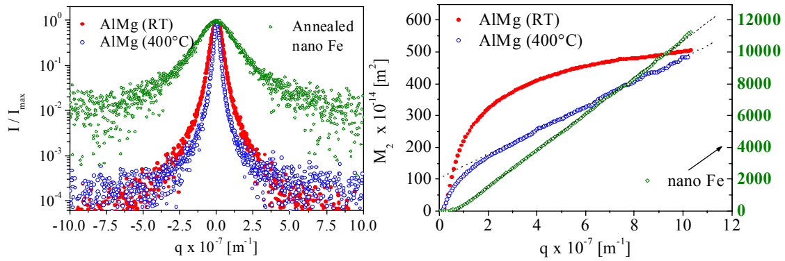
Fig. II.48 : A gauche diagrammes de diffraction dans le cas d'une pure distorsion du réseau (AlMg à température ambiante RT), d'un pur effet de taille (nano Fe :poudre de fer ball mealled ? et recristallisée) et d'un effet de taille et de distorsion combiné (AlMg déformé à 400°C). A droite les moments d'ordre 2 correspondant. q est noté s dans ce manuscrit ou S - S_b
