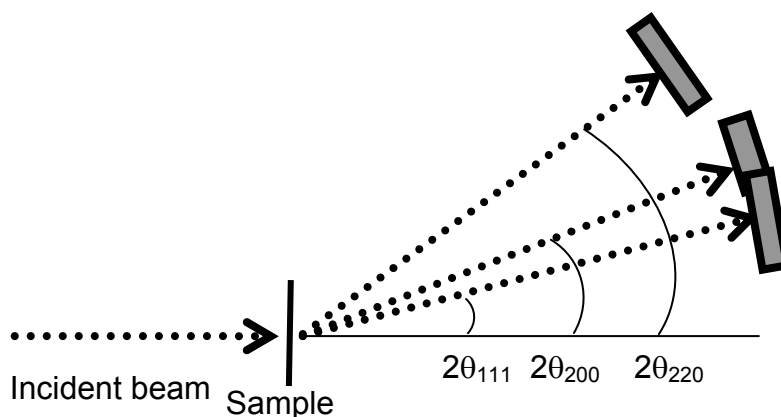
Fig. III.56 : Réunion des images CCD pour construire un spectre continu
