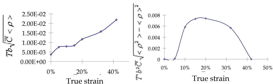
Fig. IV.68 : Evolution du paramètre de distorsion moyen et du paramètre de distorsion quadratique
