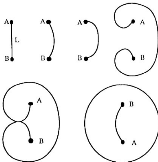
Fig. I.4 : Source de Franck et Read. La dislocation est soumise à une force par unité de longueur croissante \tau b (François et al. , 1991b)
