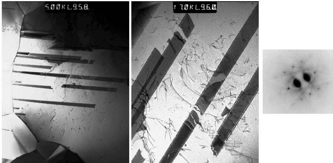
Fig. I.22 : Micrographies d'un acier Fe22.6Mn0.6C recristallisé avec une EFE de 18\text{mJ.m}^{-2} (Wang, 2008) (Mc Master University)
