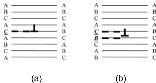
Fig. I.11 : Représentation schématisque d'une faute intrinsèque (a) et extrinsèque (b) (ALLAIN, 2004)
