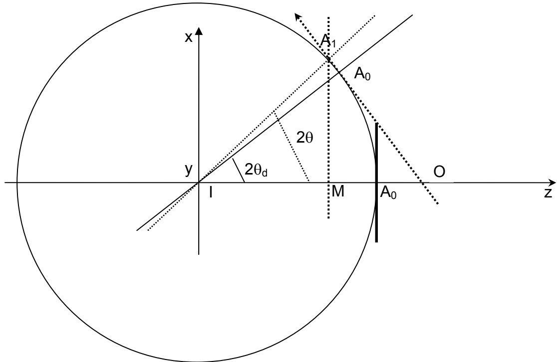
Fig. 143 : Schéma simplifié de la géométrie goniomètre / détecteur. A_0 marque la position du centre de la caméra lorsque celle-ci est à l'angle 2\theta_d . A_1 est la position du point considéré sur la caméra CCD pour ce même angle. I est l'origine du goniomètre et O est la position virtuelle du faisceau direct sur la caméra CCD à l'angle 2\theta_d
